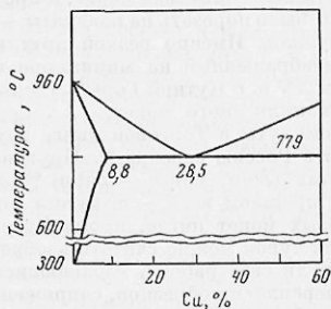
Рис. 3. Диаграмма состояния сплавов серебра с медью
