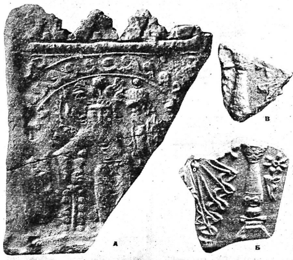
Рис. 1. Фрагменты лицевой стенки оссуария из Иштихана.
