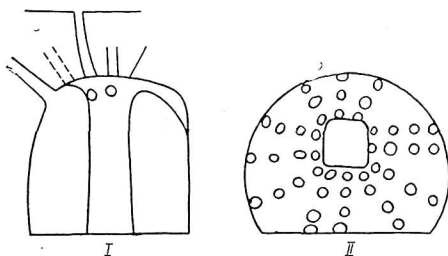
Рис. 1. Гончарная печь с Бауртепа. I — разрез, II — план свода топки.
