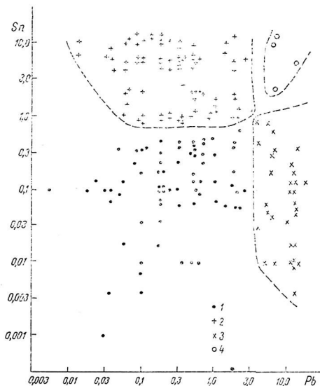
Рис. 2. Корреляционный график взаимозависимости концентраций олова и свинца в сапаллитенинских медях (по данным 194 анализов).
