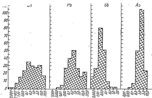
Рис. 1. Гистограммы распределения концентраций олова, свинца, сурьмы и мышьяка в сапаллитепинской меди (по данным 194 анализов).
