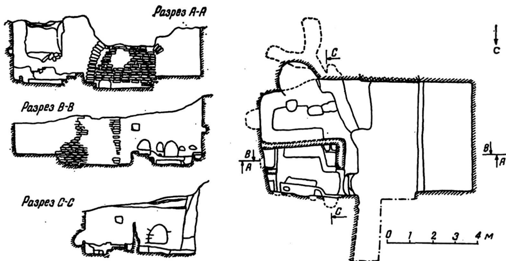
Рис. 1. План и разрезы помещения.
