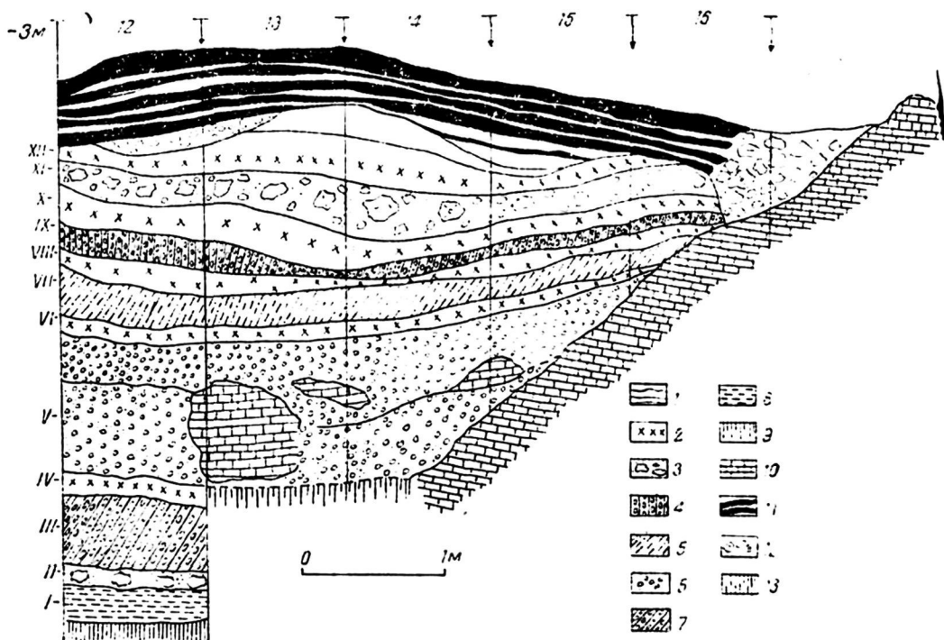
Рис. 1. Стратиграфия нижнепалеолитической пещерной стоянки Сель-Унгур.
