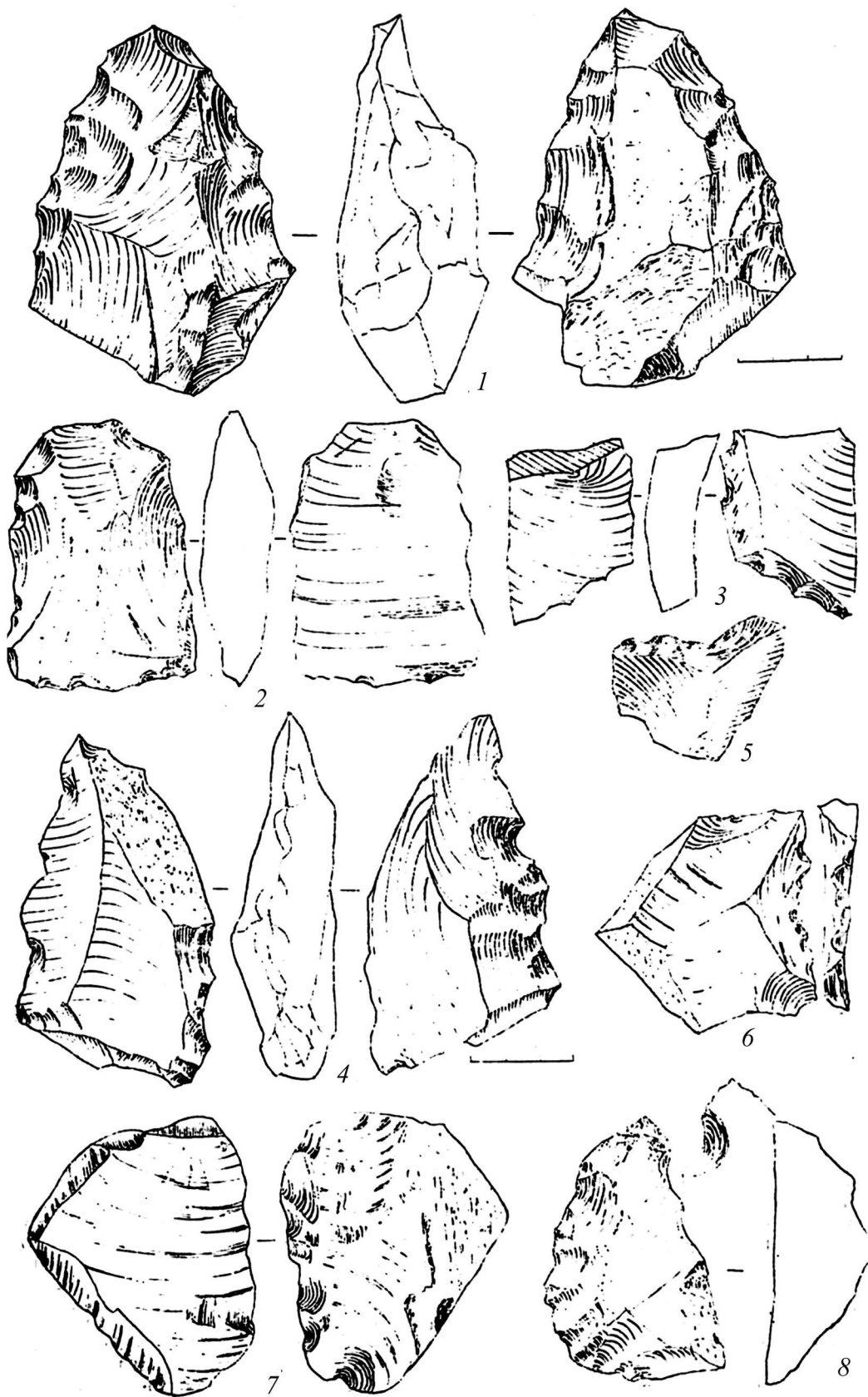
Рис. 2. Виды каменных орудий из пещерной стоянки Сель-Унгур.
