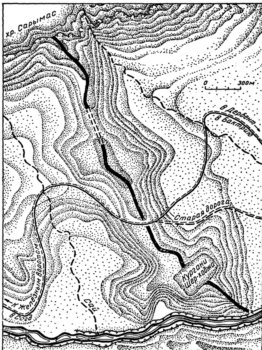
Рис. 2. План кушанской пограничной стены у к. Дербент.
