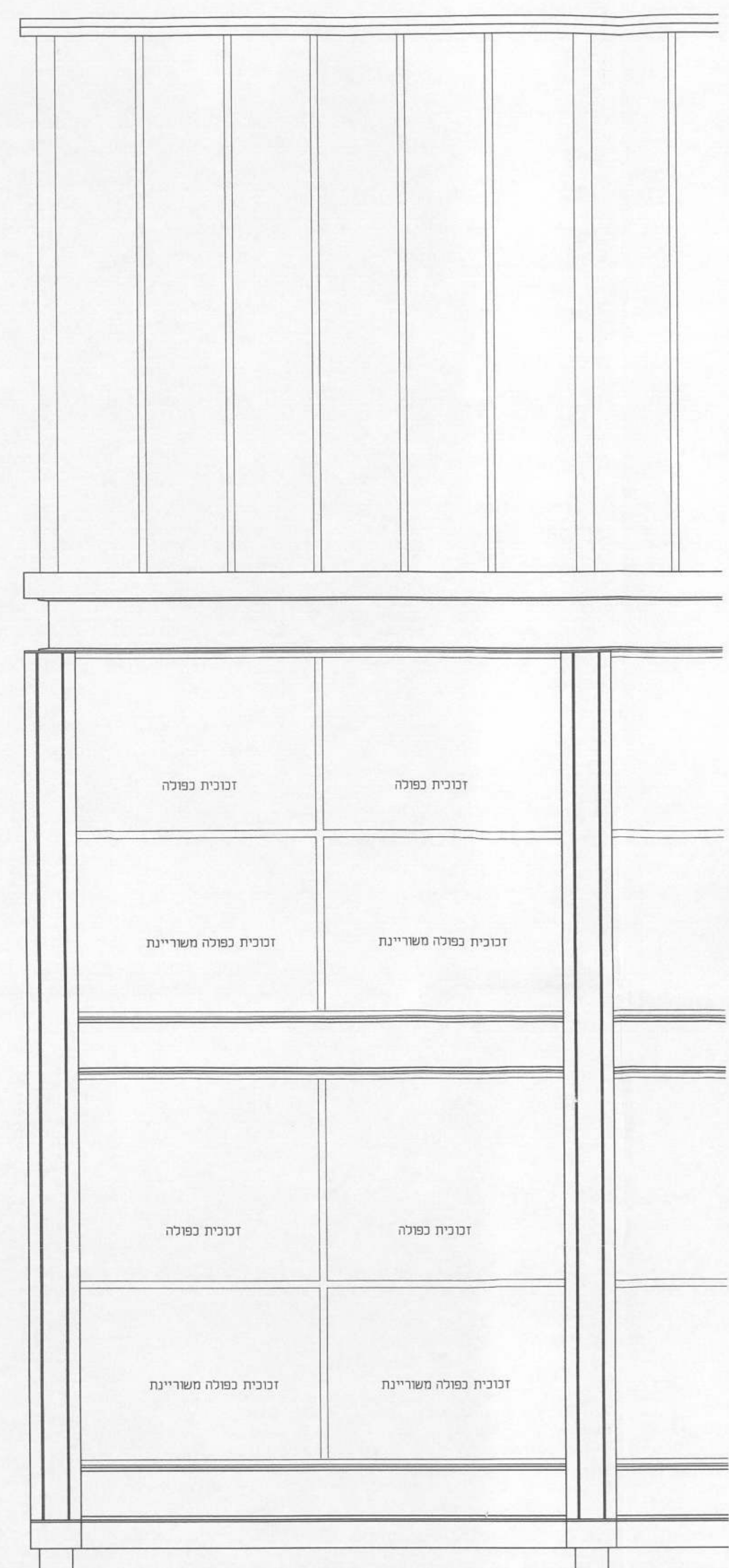
קטע חזית עם חלוקת הזכוכית בכל מודול ק.מ. 1:20
