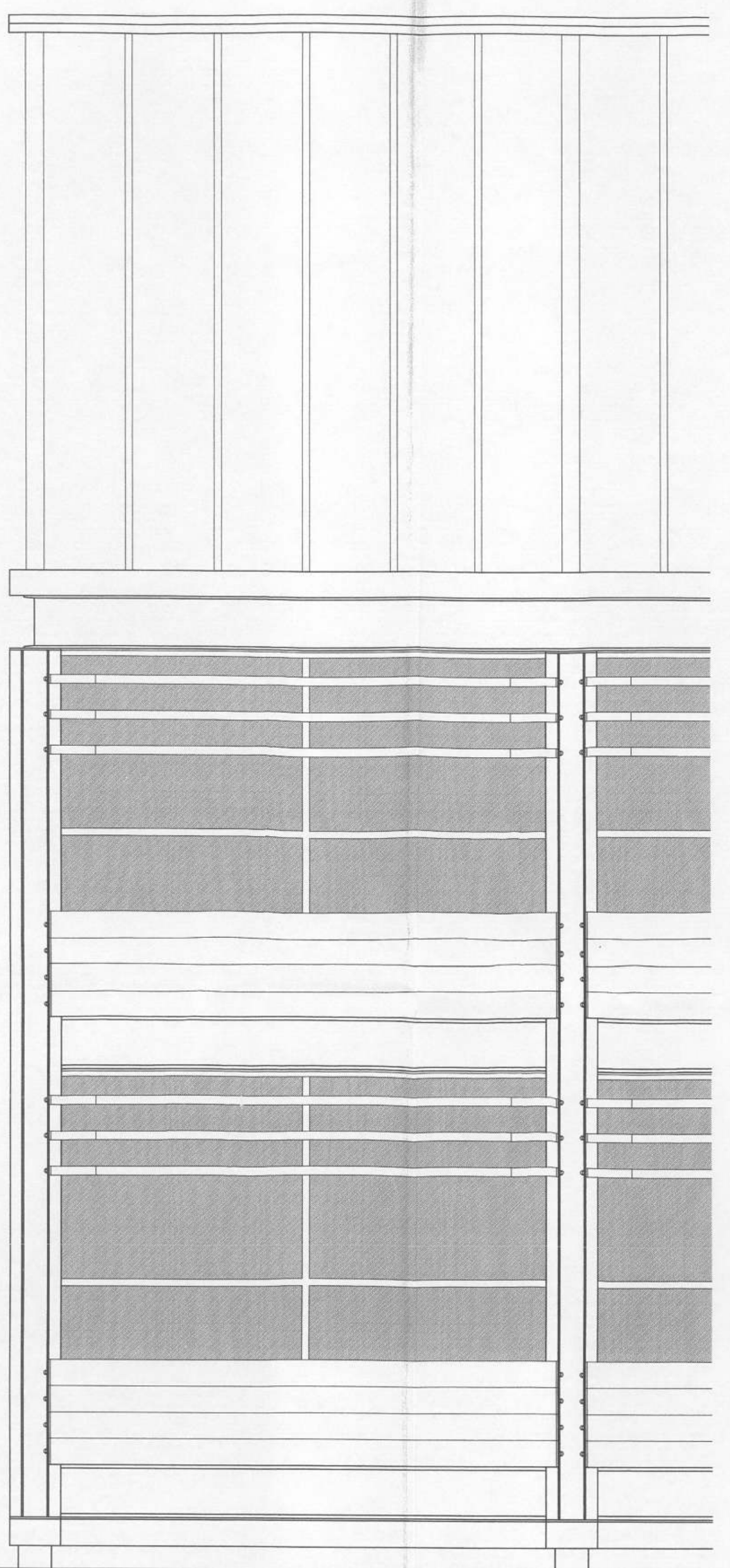
קטע חזית עם אלמנטי הצללה ק.מ. 1:20
