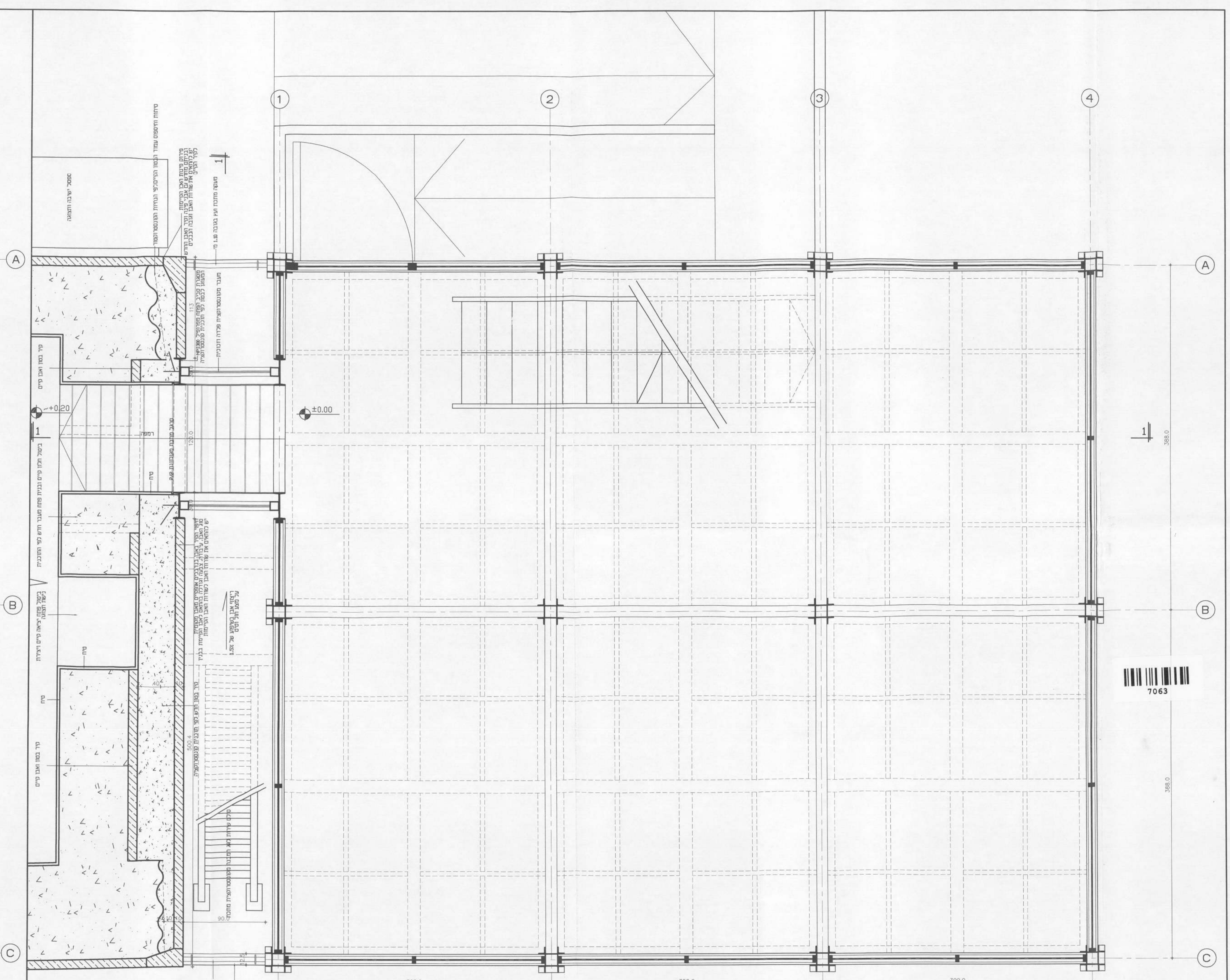
תוכנית קומת קרקע
