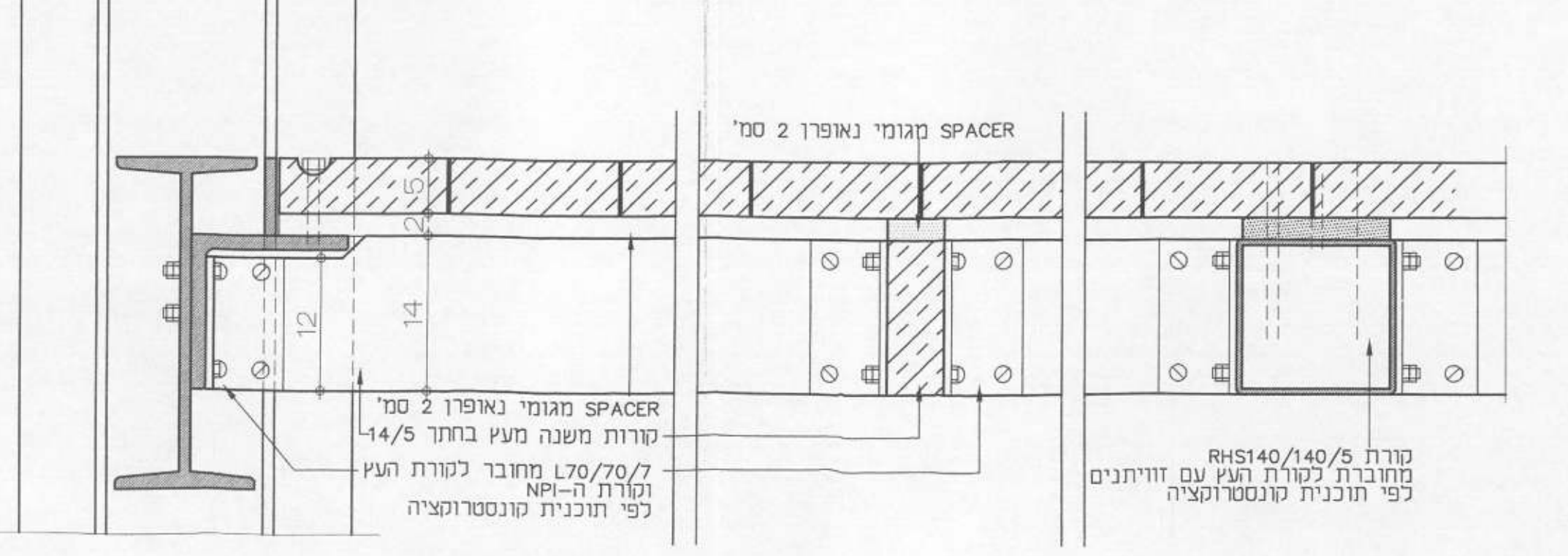
חתך 2-2 15
