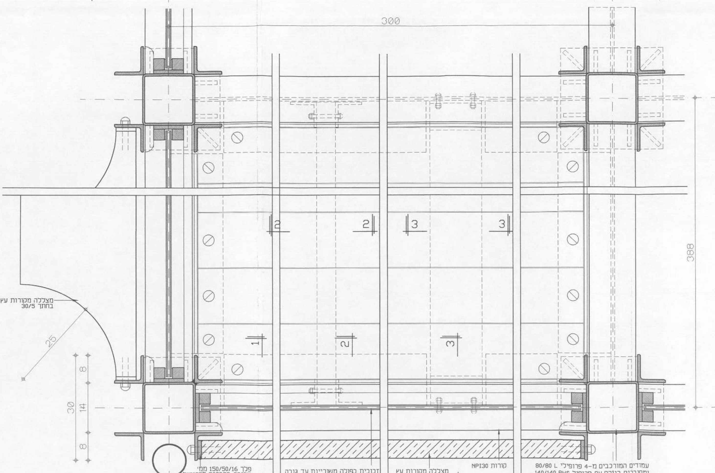
חתך אופקי של שדה טיפוסי בבנין ק.מ. 1:5
