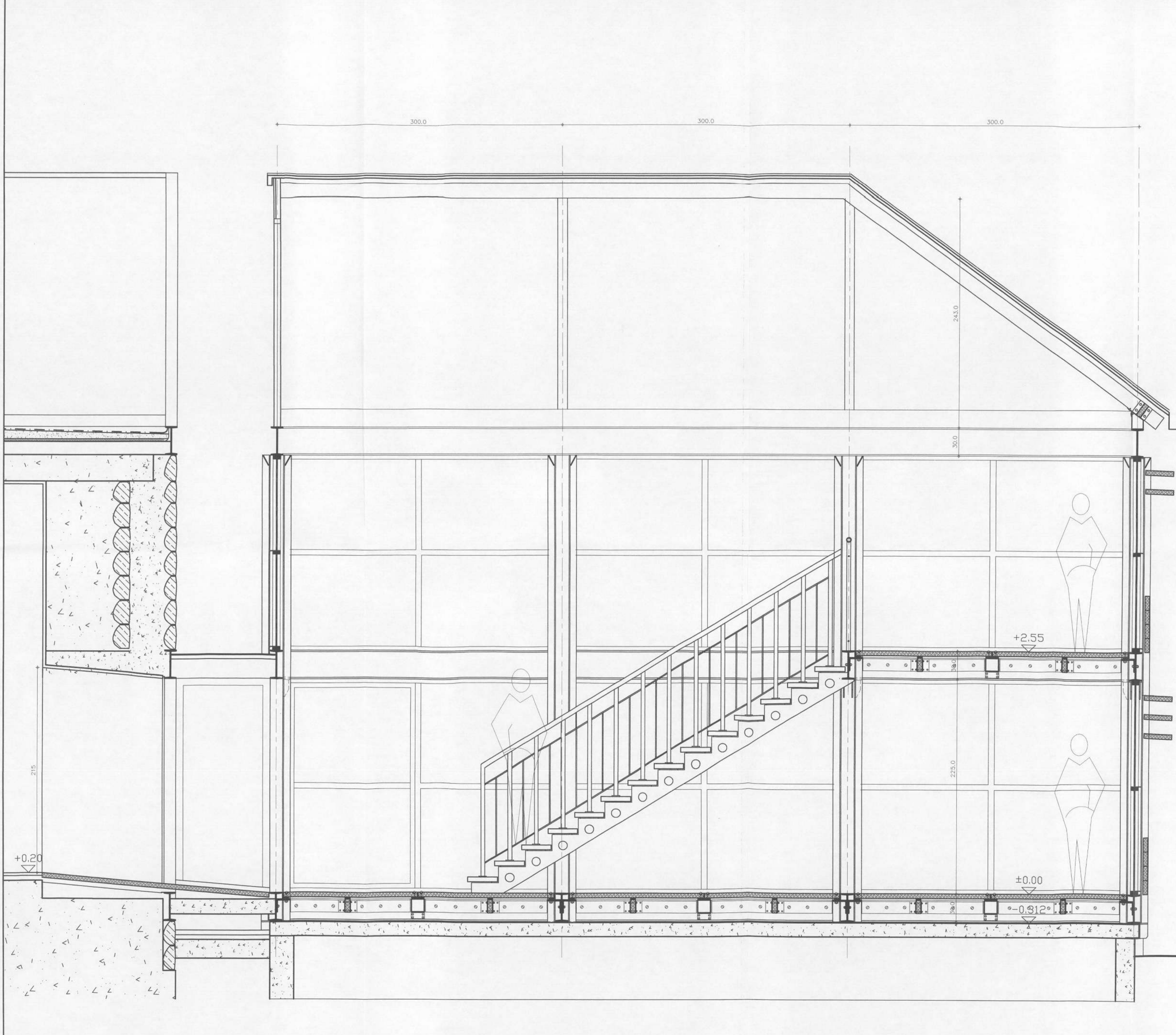
חתך אורך 1-1
