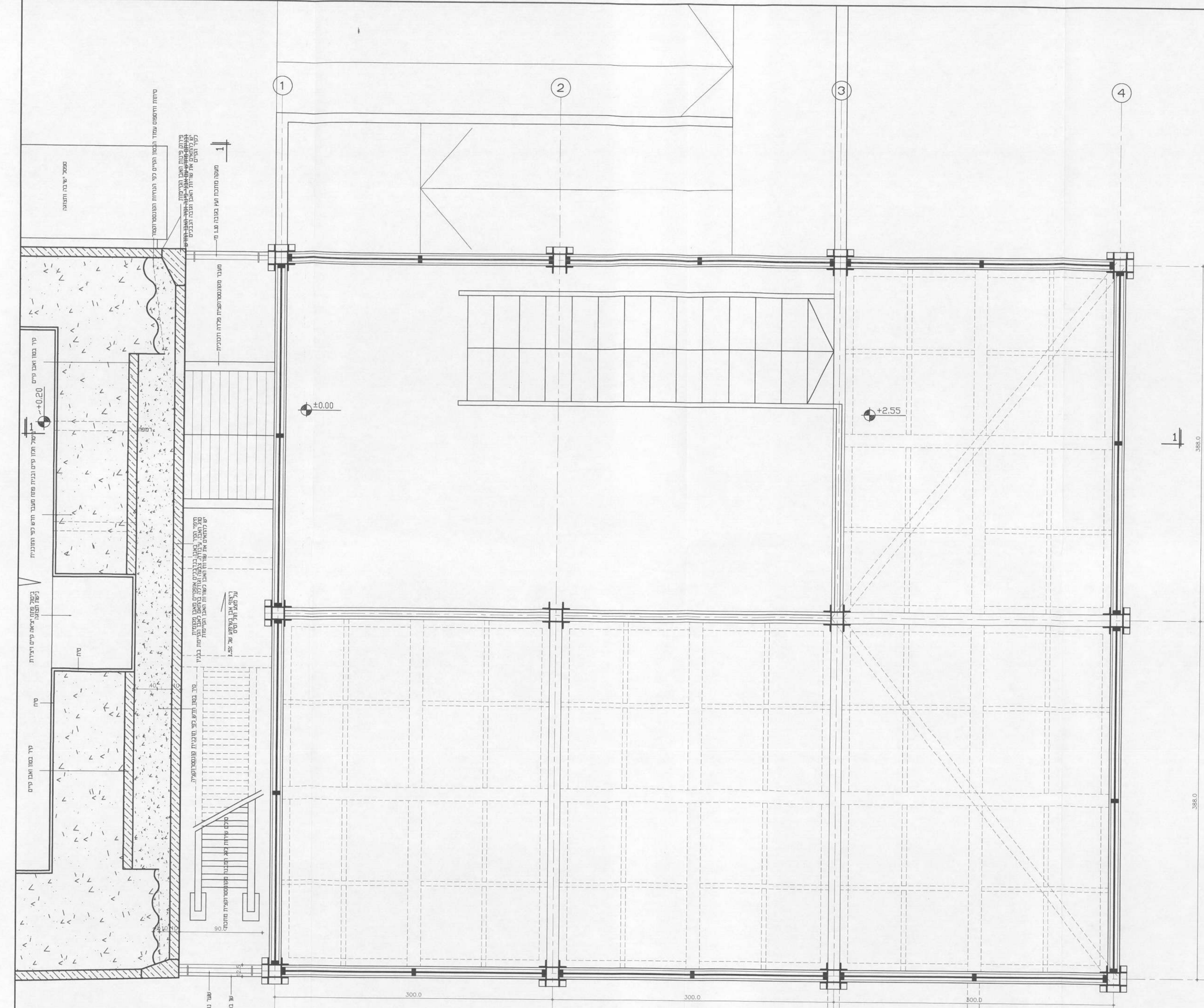
תוכנית קומה גלריה
