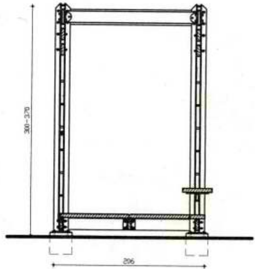
חַתָּךְ רוּחֵב
