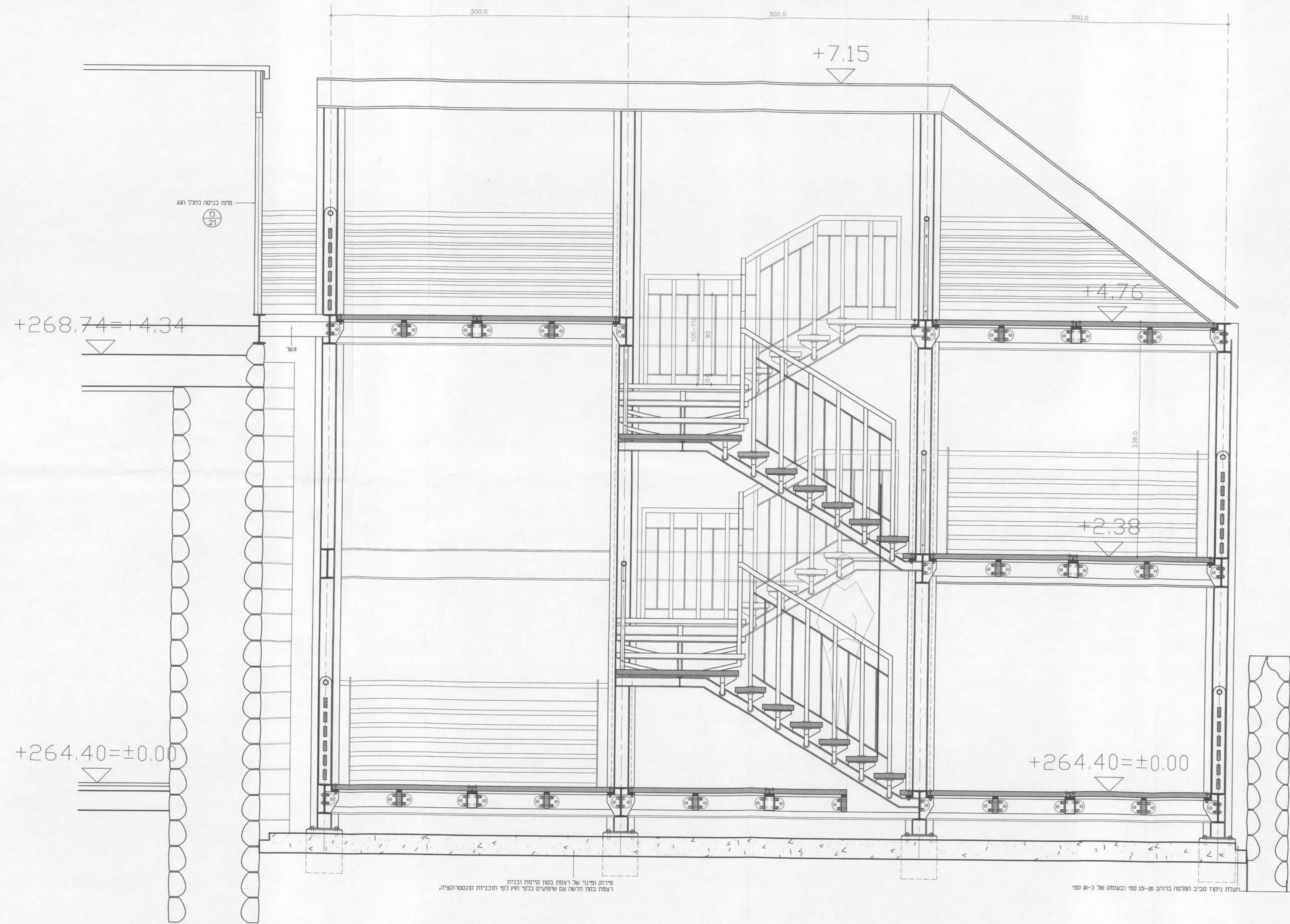
חתך 1-1
