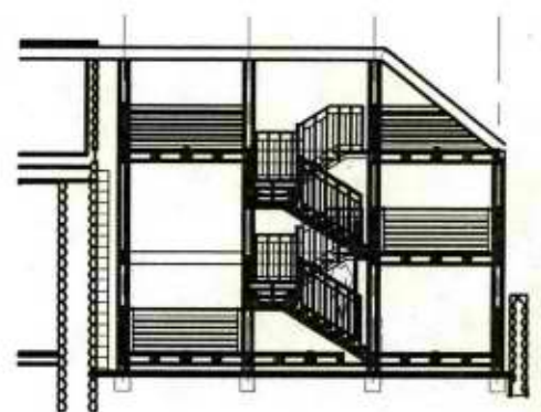
חתך אורך
