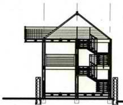
חתך רוחב
