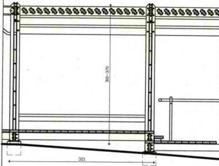
חַתָּךְ אֹרֵר
