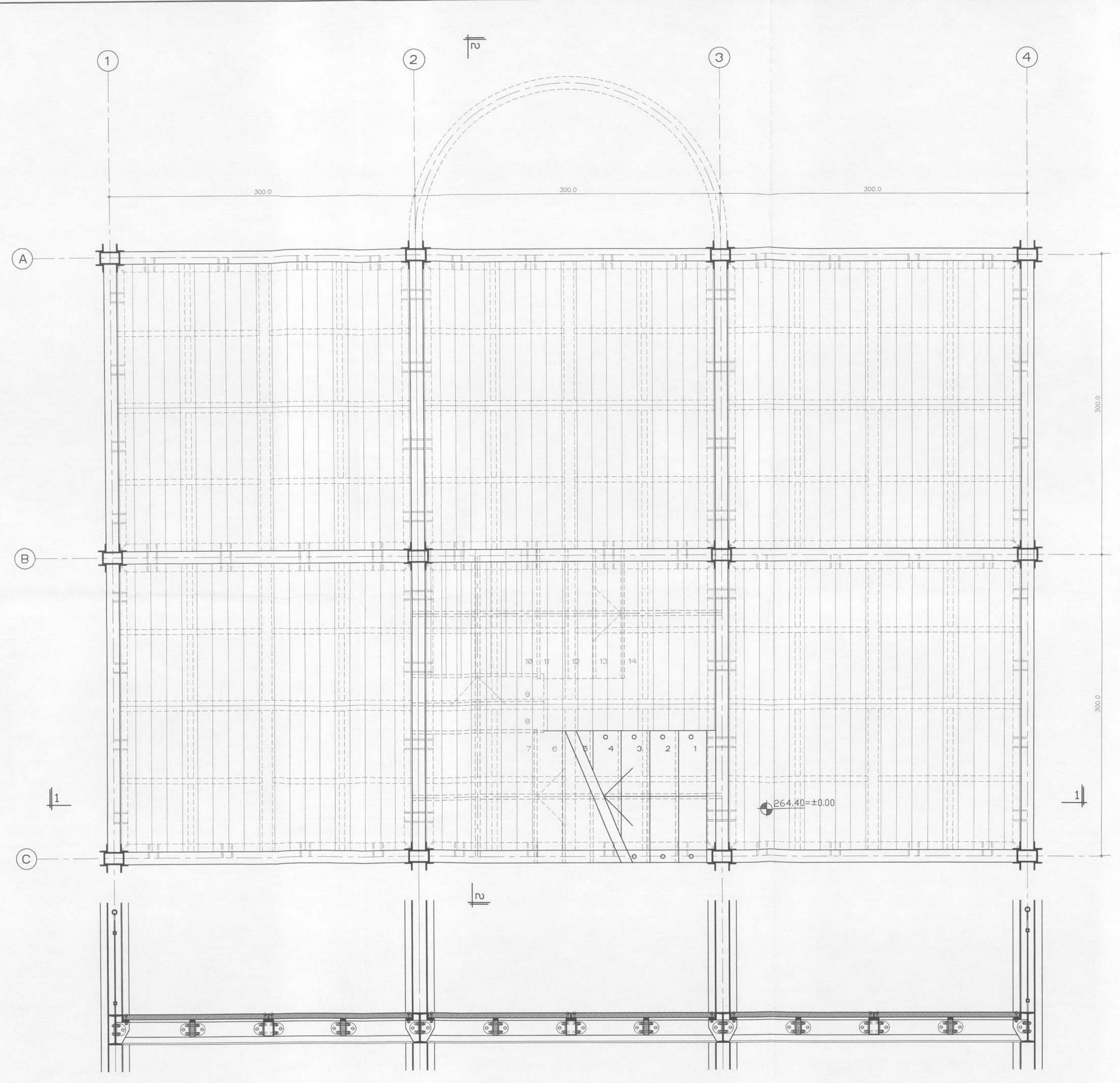
תוכנית קומה קרקע וחתך בתקרה/רצפה
