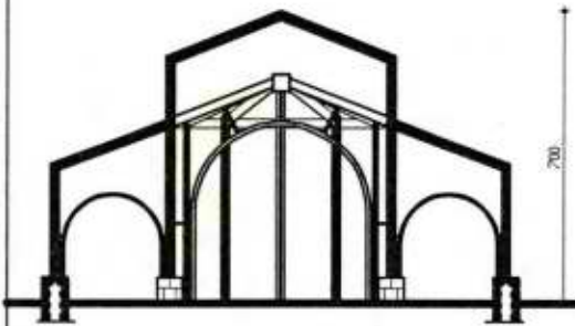
חתך רחב
