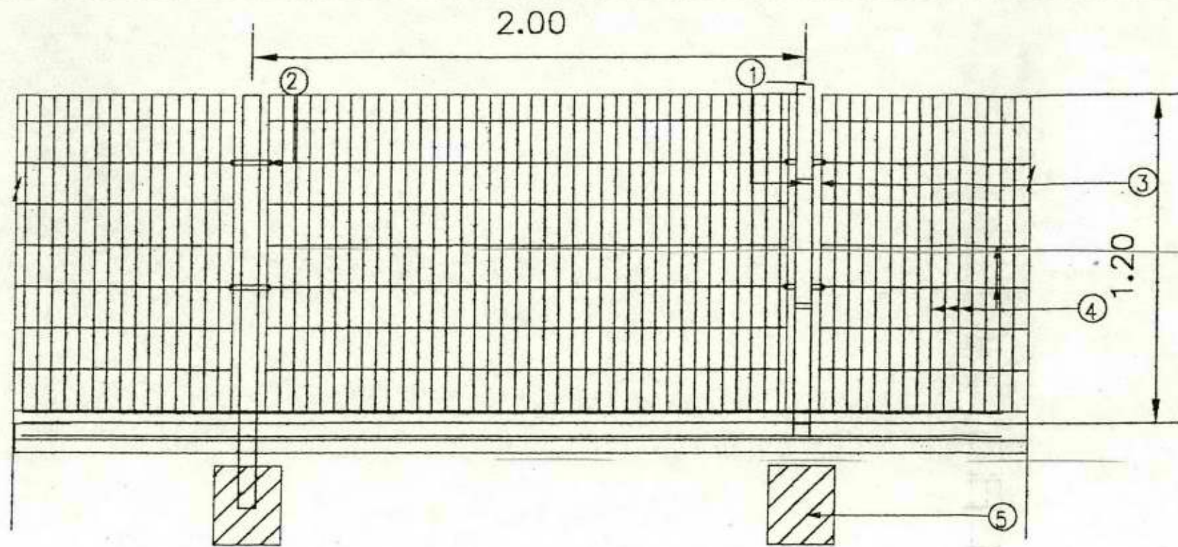
חזית ק.מ. 1:20
