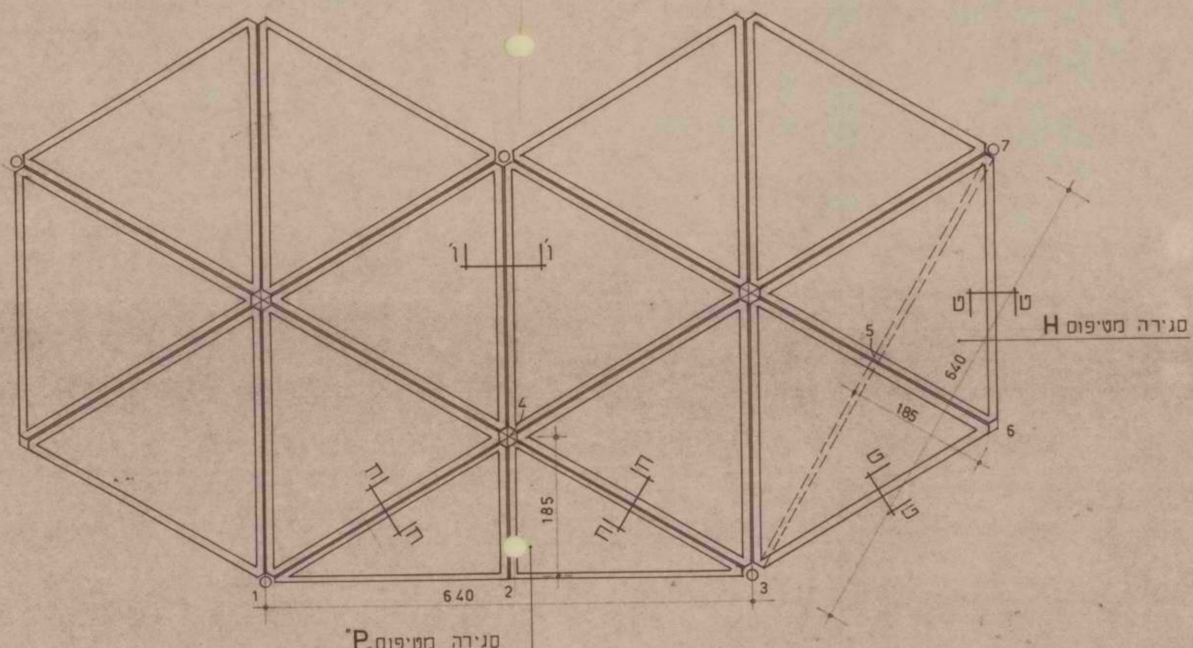
סגירה מטיפוס H חיבור בין הסככות וטיפוסי סגרות עי הפנלים מבט מלמעלה ק.מ. 1:50
