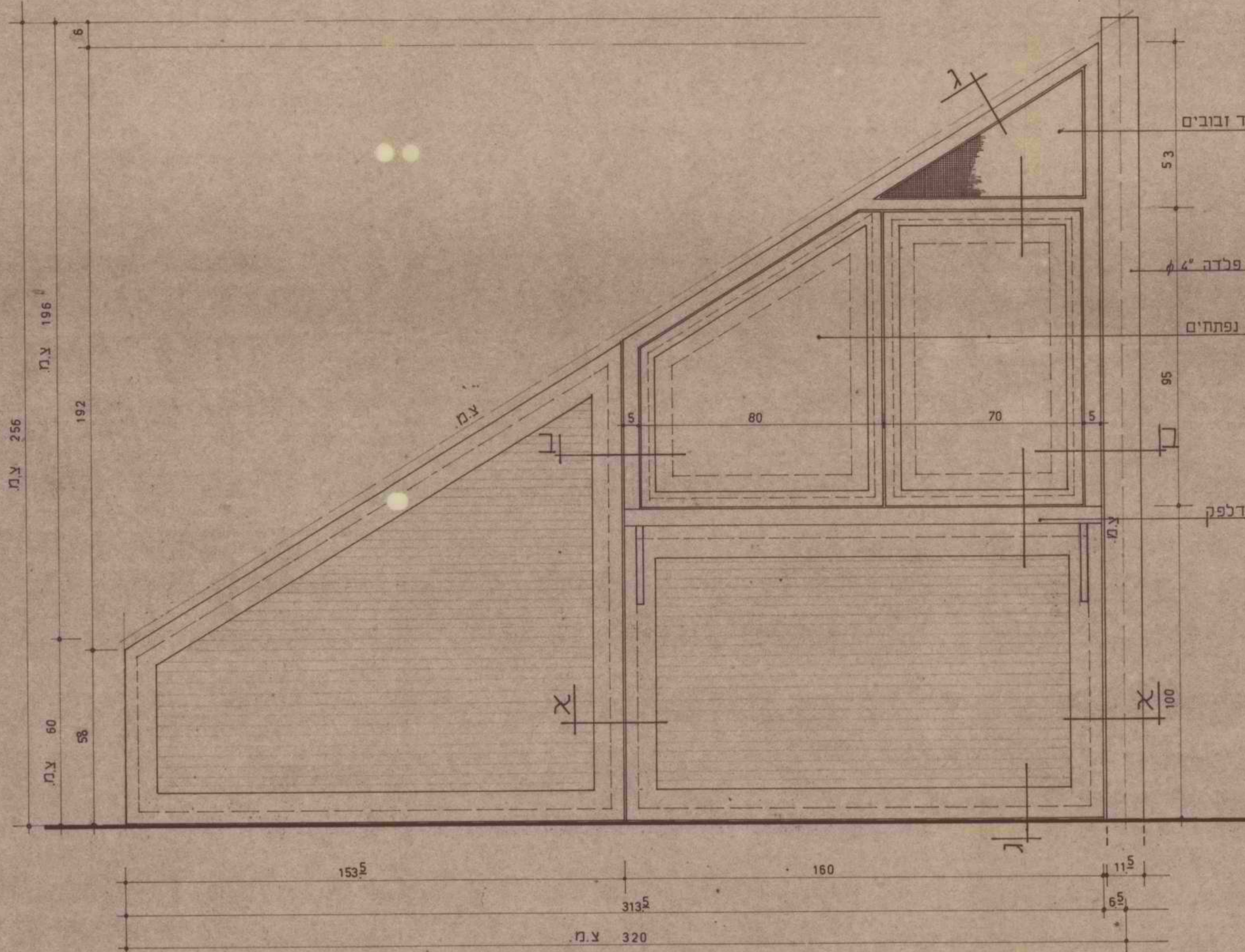
פנל מסיפוס W הבא במקום פנל S במשרד ומלתחות ק.מ. 1:10 כמות במיבנה * 4
