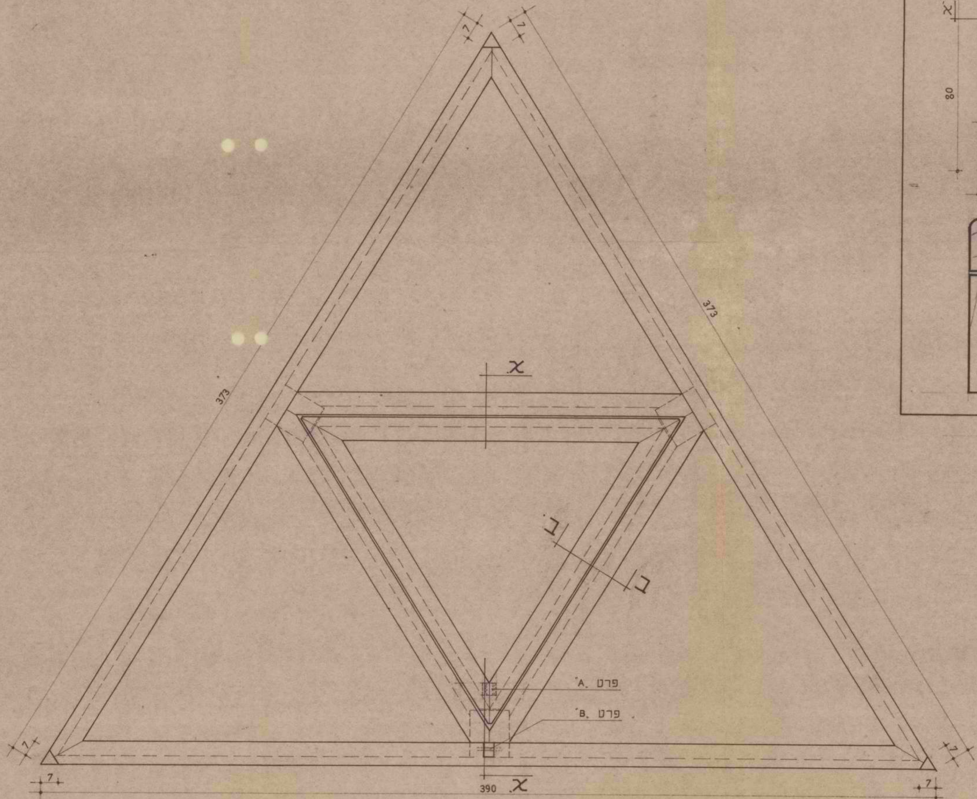
פנל R במידות כמו פנל נא' ובנוי כמוהו (ראה תכנית קונסטרוקציה מס' 507/5) כאשר בתוכו מורכב חלון קנדקס. המיקום המדויק של פנל R' ראה בתכנית הגג. ק.מ. 1:10
