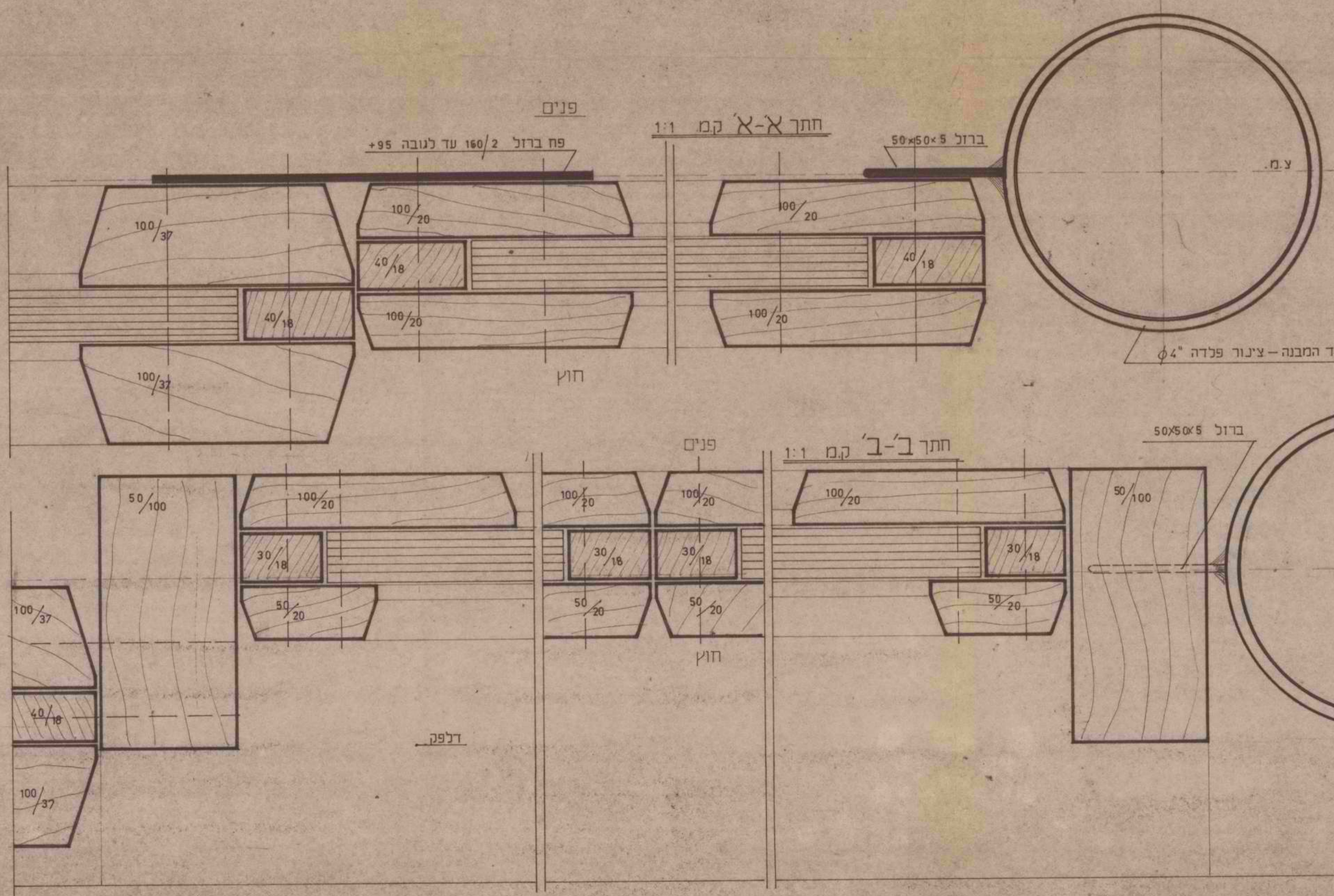
פנל מסיפוס W הבא במקום פנל S במשרד ומלתחות ק.מ. 1:10 כמות במיבנה * 4
