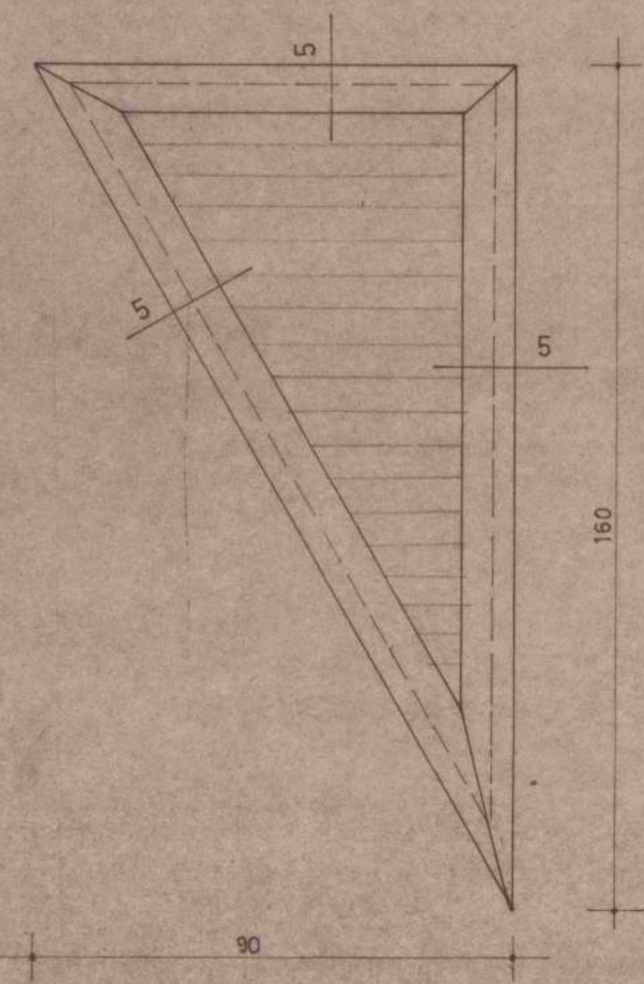
פנל סגירה צ קמ 1:20
