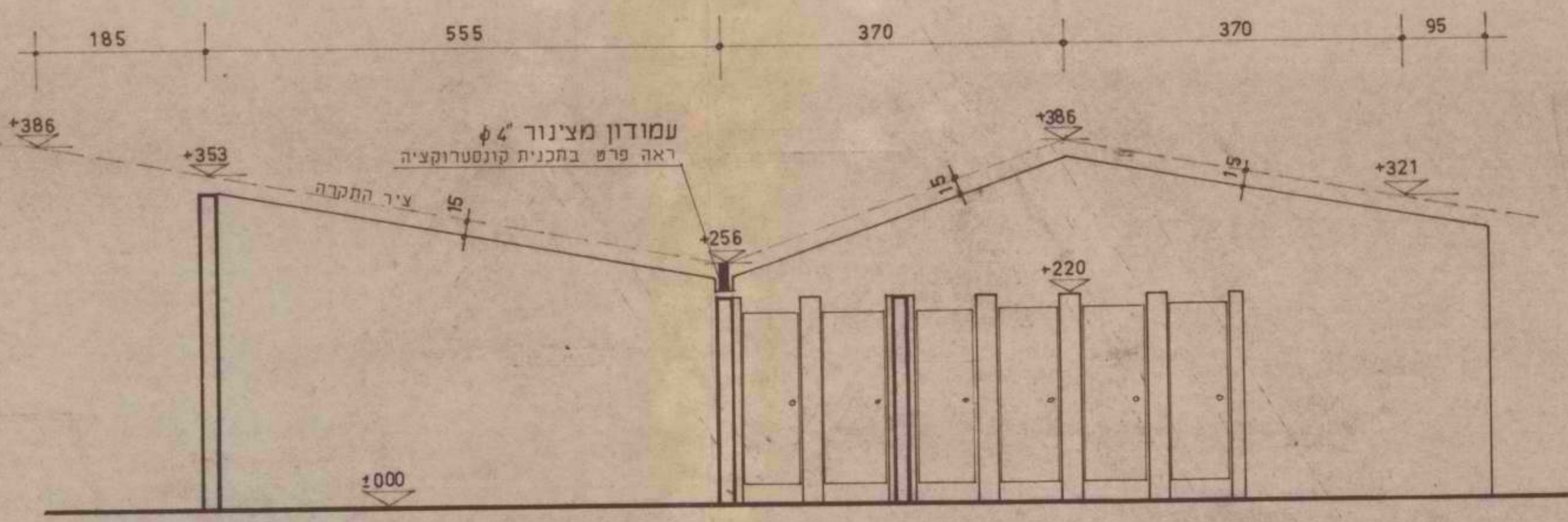
חזית הקיר המפריד בין מקלחות ו-4 גברים לבין מקלחות ו-4 נשים גובה הקיר, לכל אורכו, -16 מפני התקרה (ציר התקרה) ק.מ. 1:50
