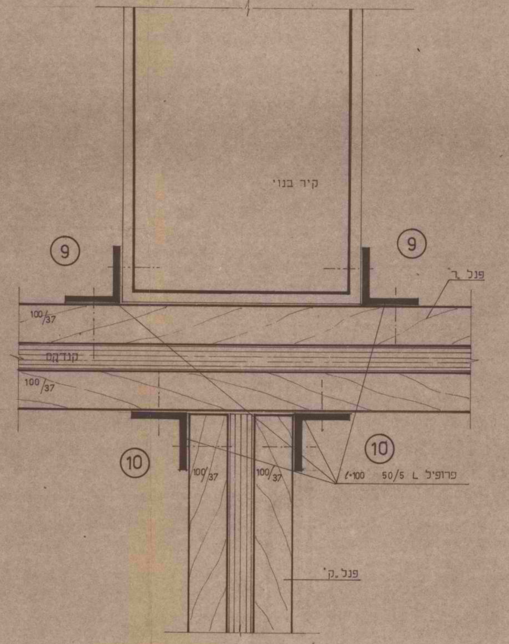
פרט חיבור פנלים ג,ק קמ 1:2
