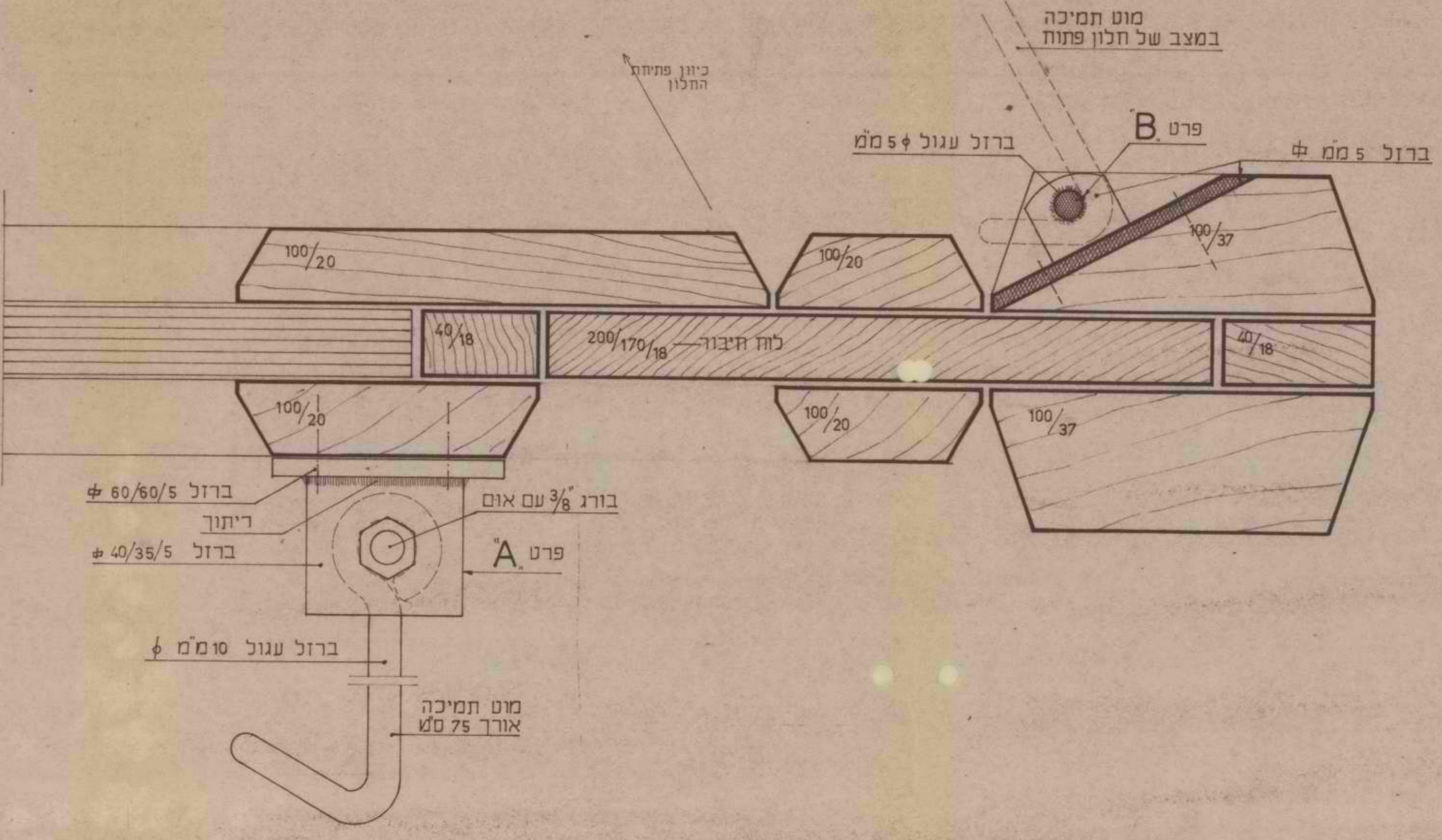
פנל R במידות כמו פנל נא' ובנוי כמוהו (ראה תכנית קונסטרוקציה מס' 507/5) כאשר בתוכו מורכב חלון קנדקס. המיקום המדויק של פנל R' ראה בתכנית הגג. ק.מ. 1:10
