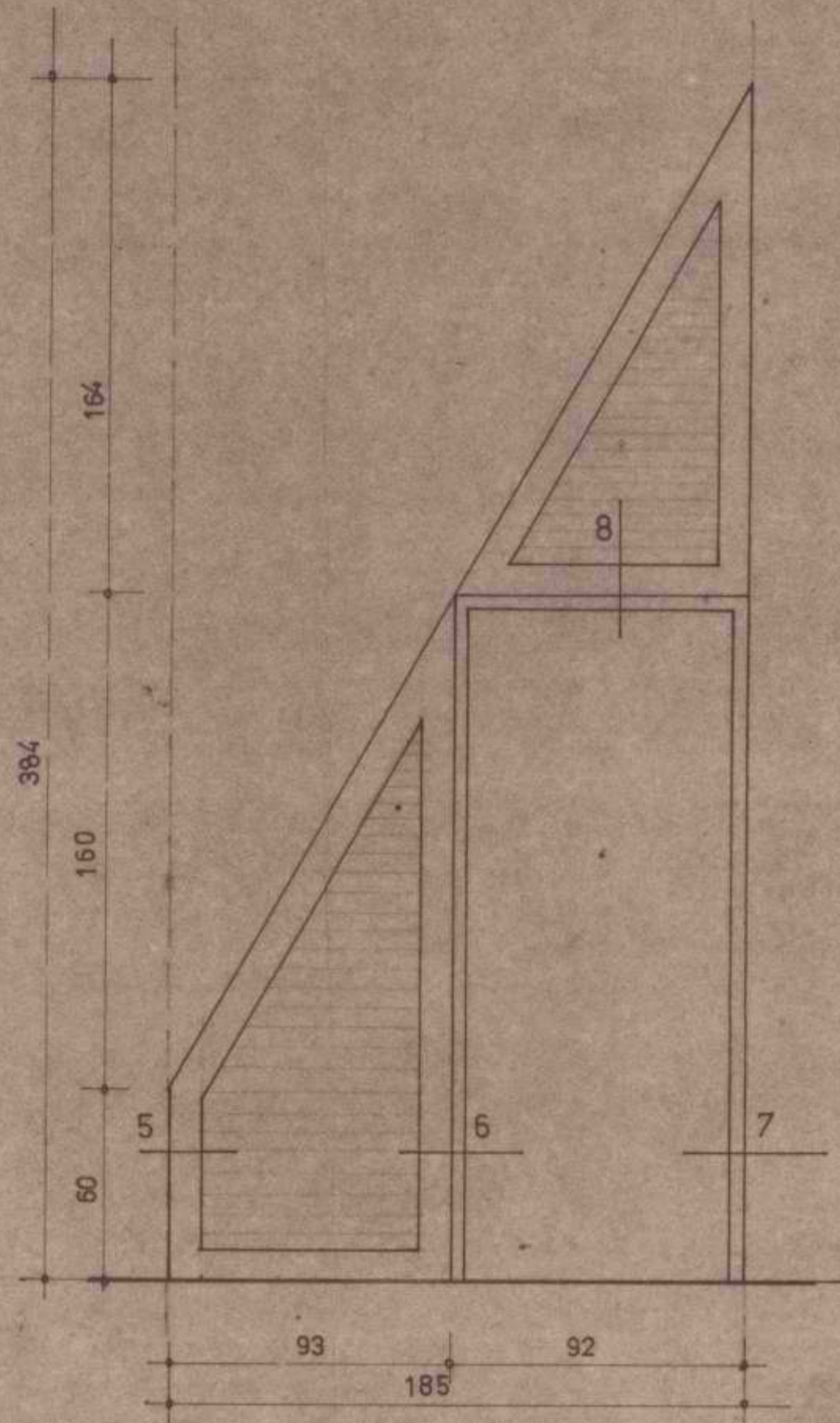
פנל סגירה צ קמ 1:20
