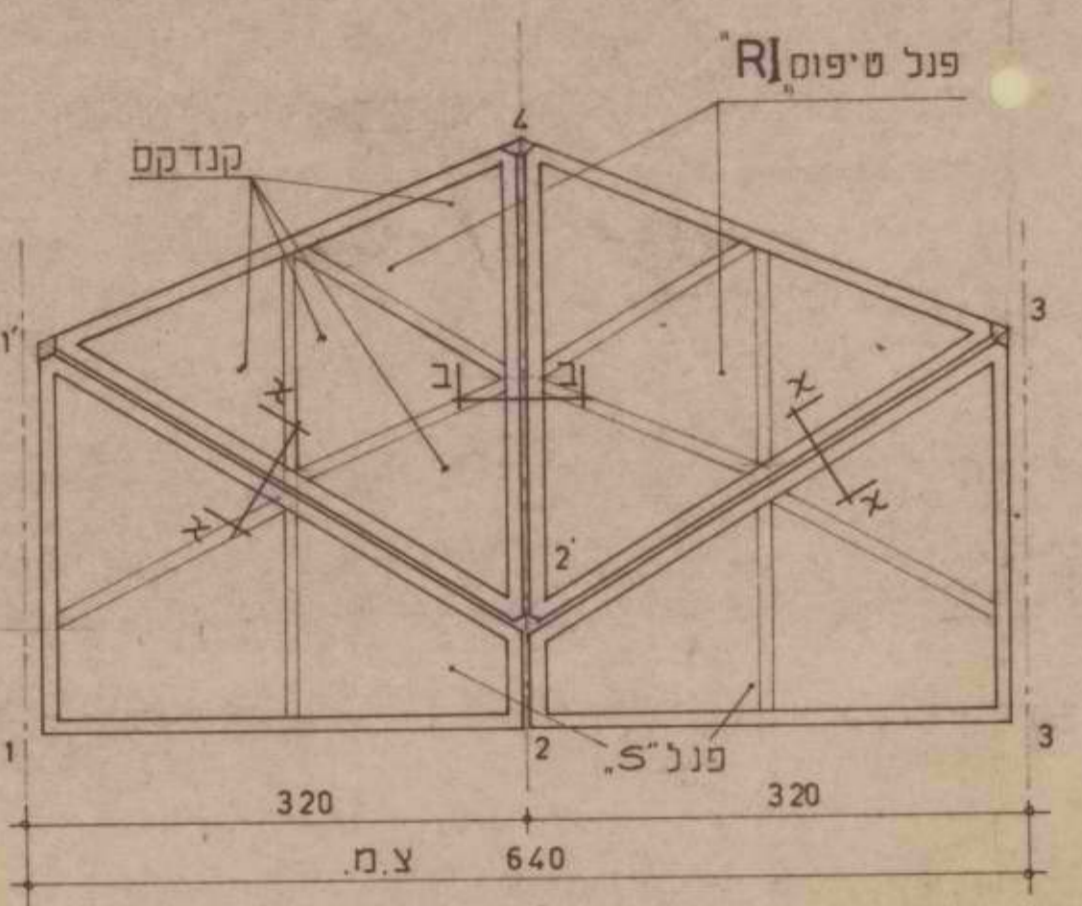
פנל טיפוס R1 סגירה מטיפוס P חזית 1-3 ק.מ. 1:50 סגירה מטיפוס H חזית 3-7 ק.מ. 1:50 (חתכים א-א, ב-ב ראה גיליון מס 501/20)
