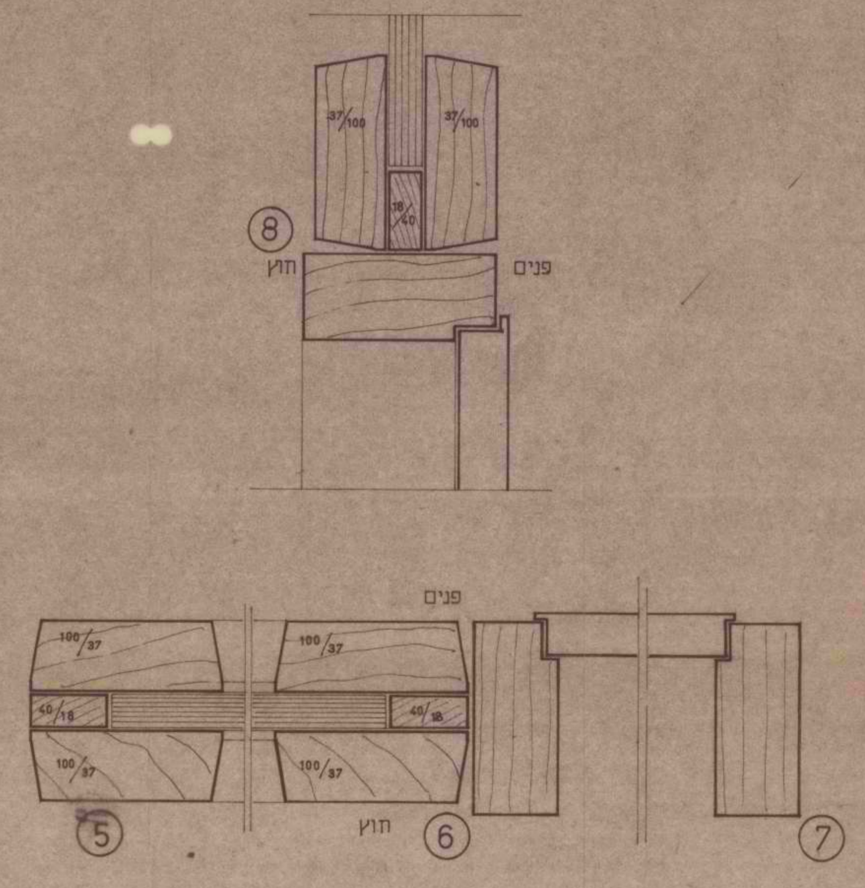
פרטי פנל צ קמ 1:2
