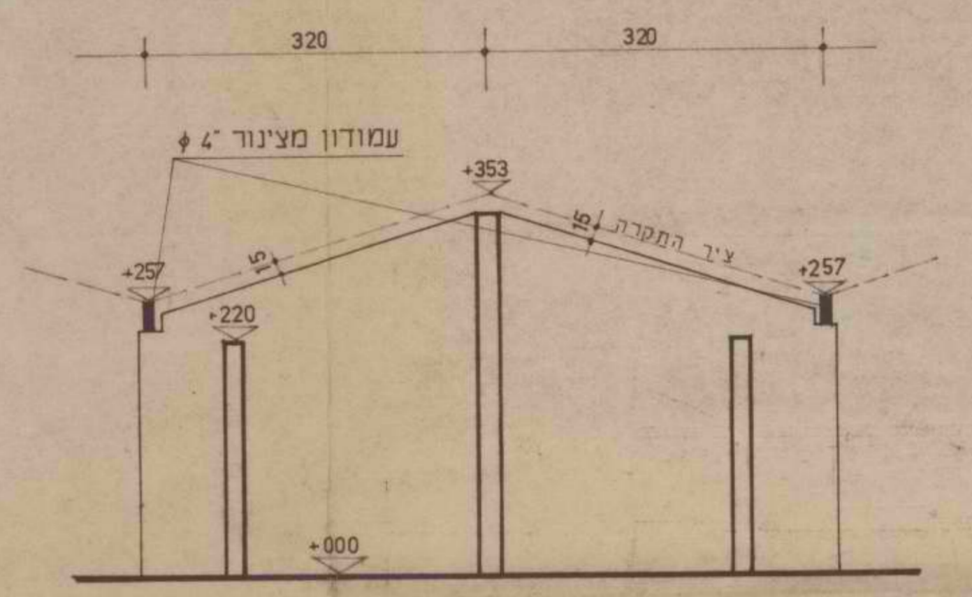
חזית הקיר המפריד בין המלחה לבין המקלחות ק.מ. 1:50
