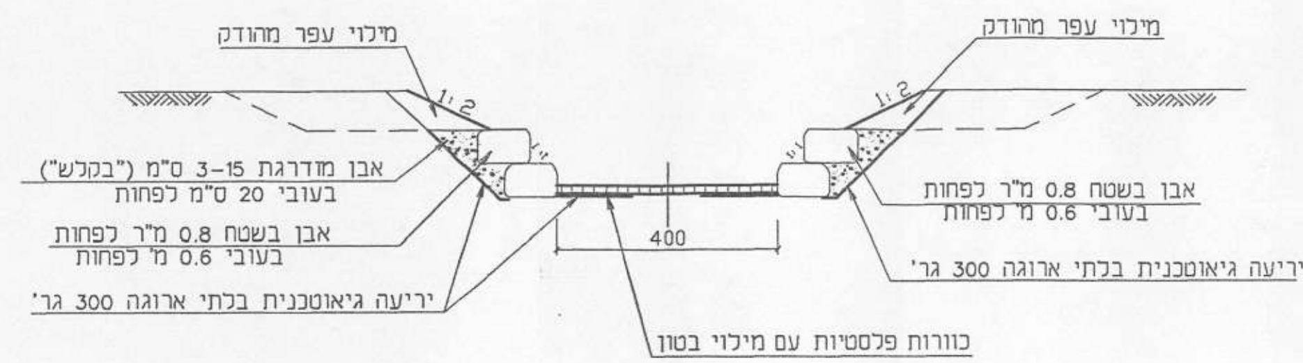
חתך 2-2 1 : 100
