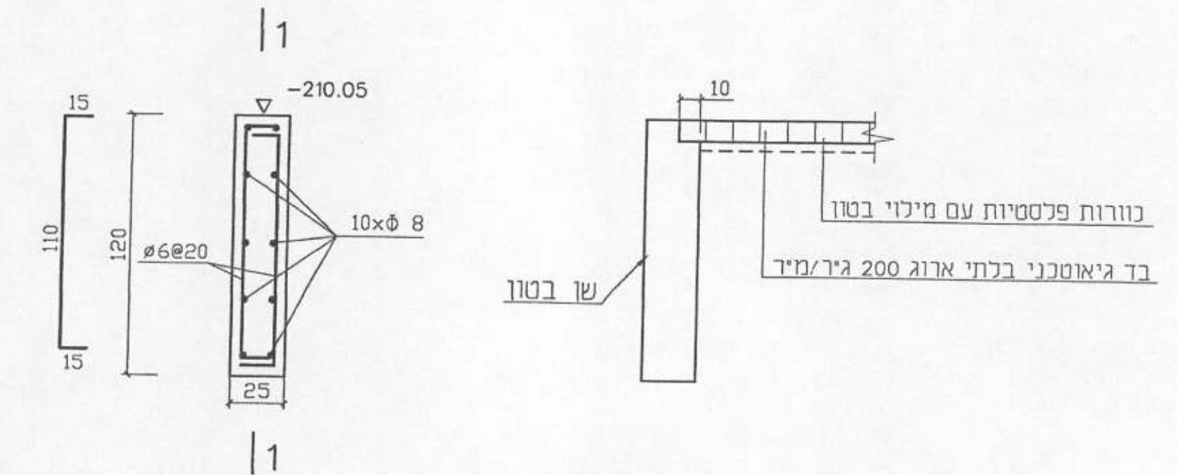
פרט שן בטון 1 : 25
