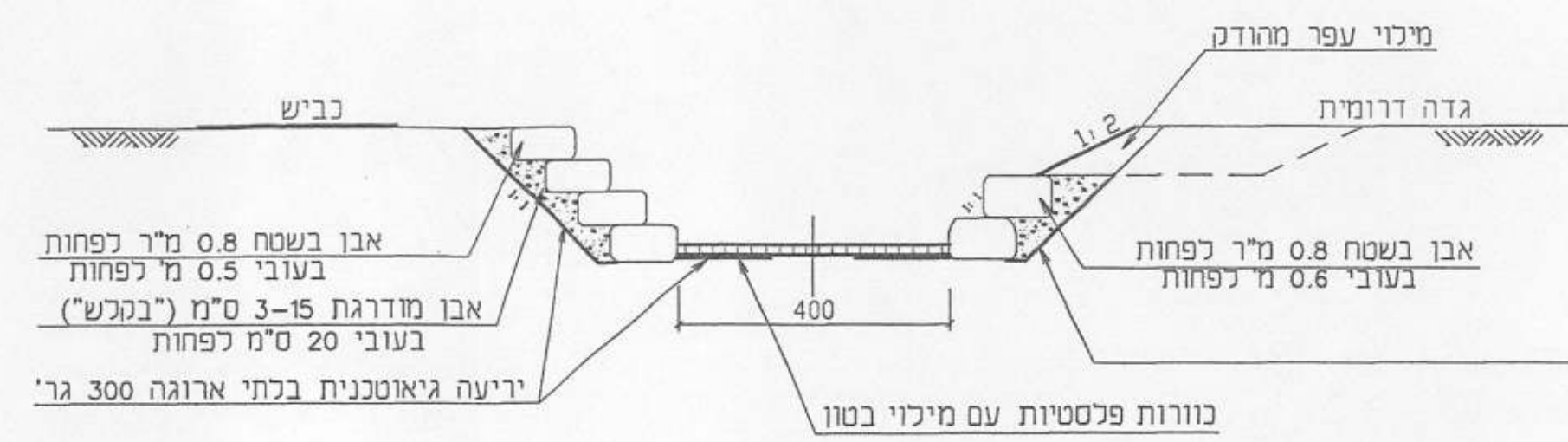
חתך אופייני 1 קטע חתכים 4 + 9 1 : 100
