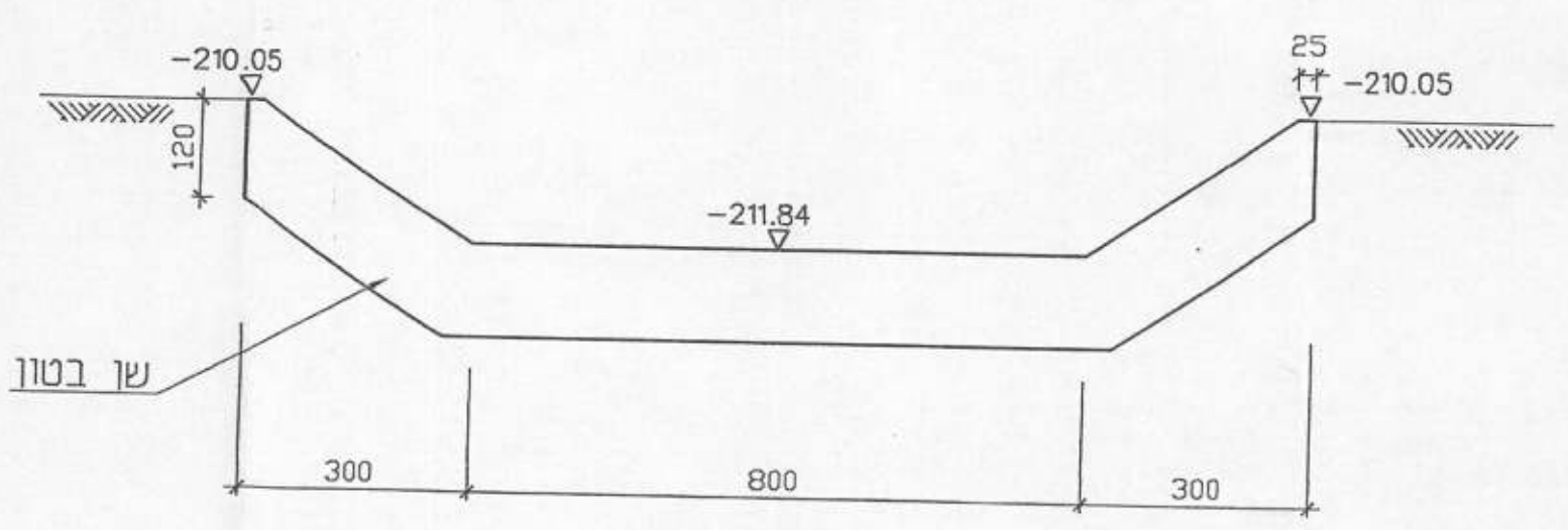
חתך 1-1 1 : 100
