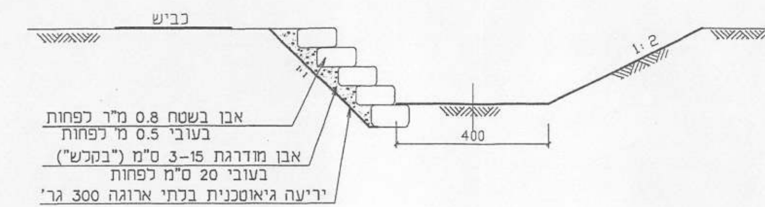
חתך אופייני 2 קטע חתכים 9 + 15 1 : 100
