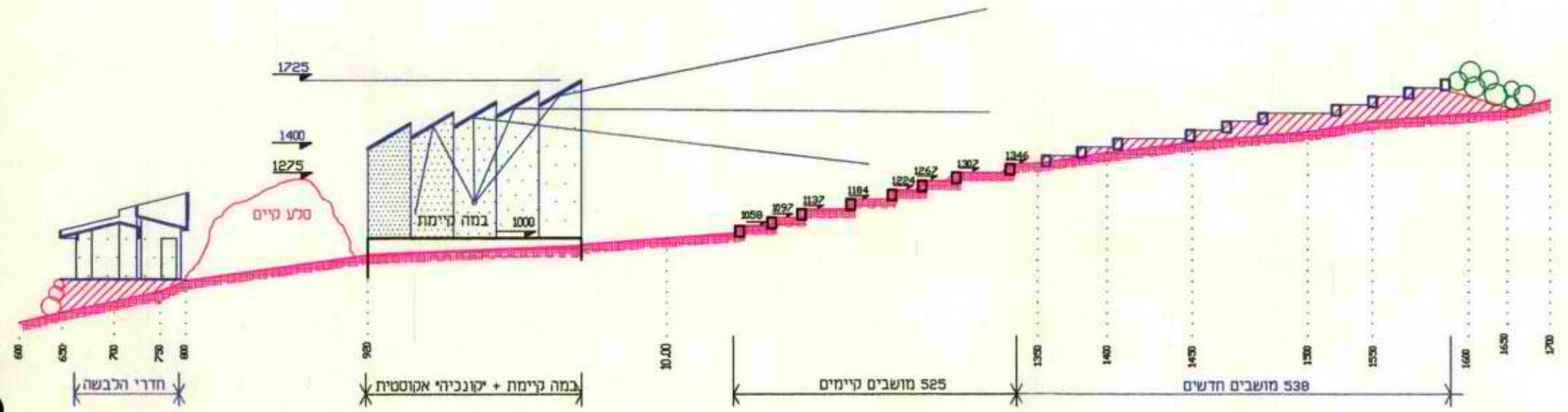
חתך עקרוני
