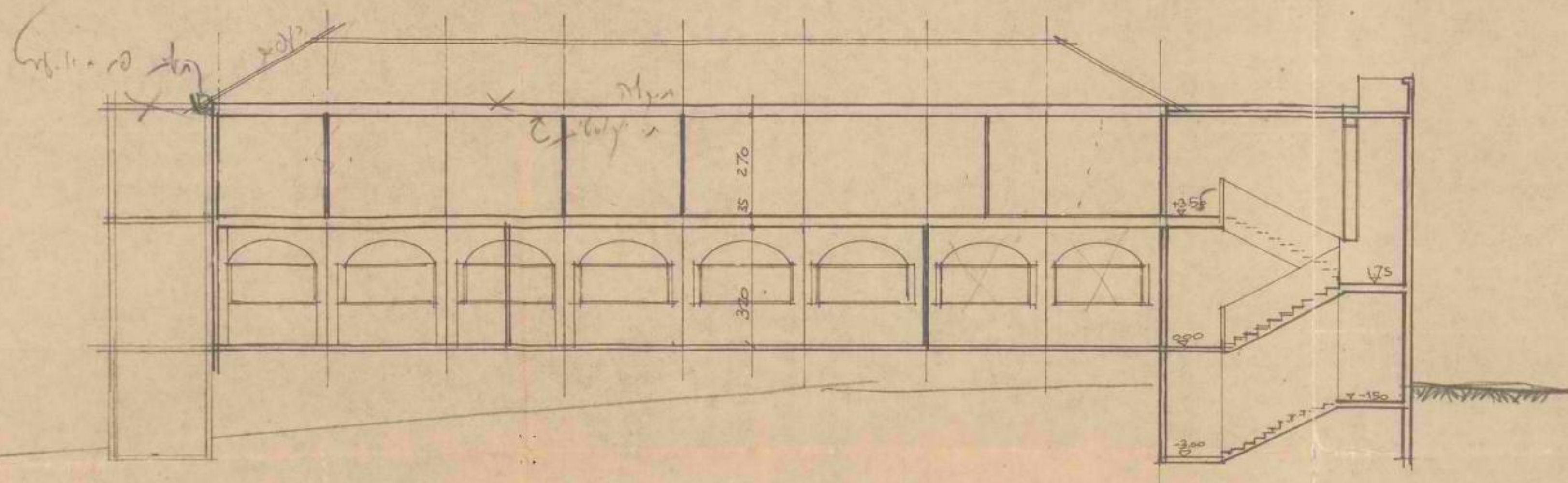
1:100 חתך ט-ט
