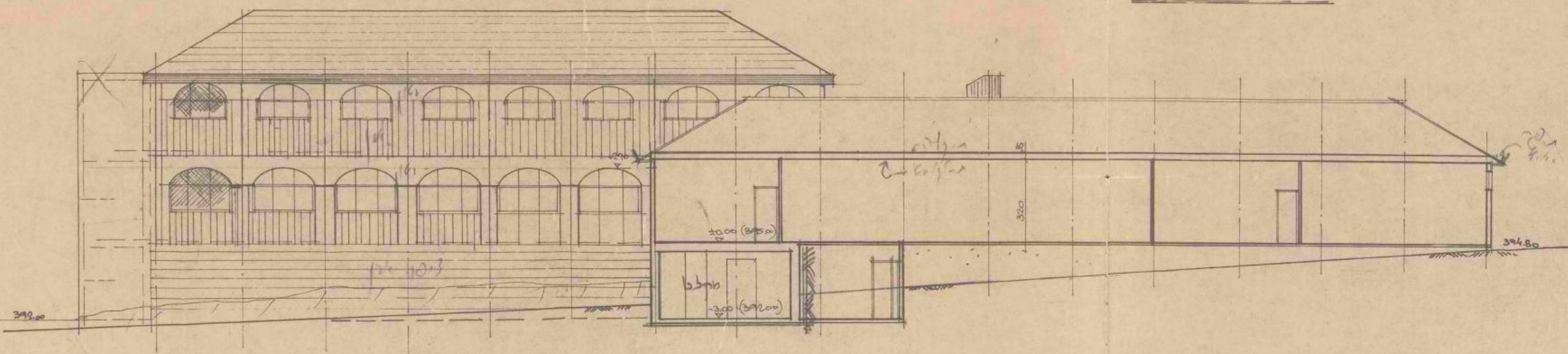
1:100 חתך מ-מ
