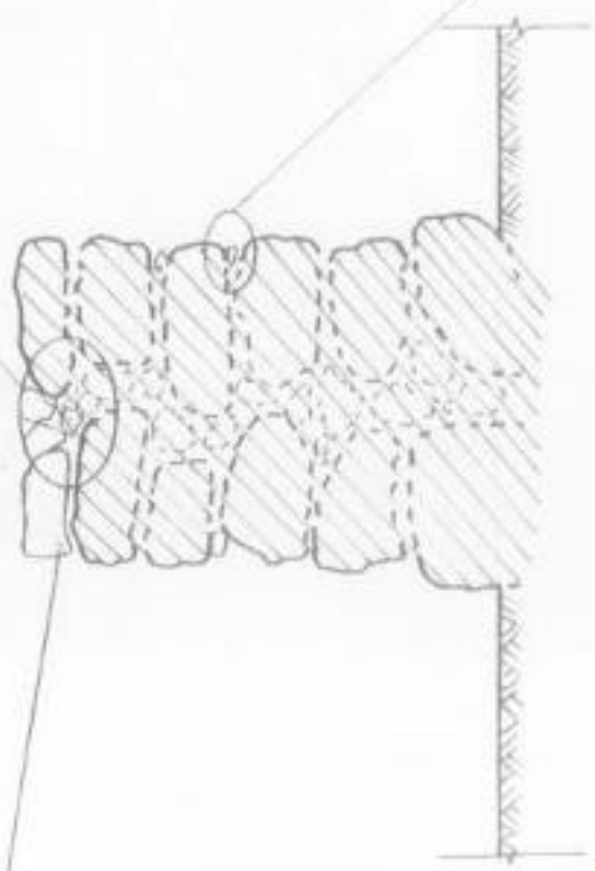
פרט 1 - עקרוני לייצוב קירות הבנויים שני פנים
