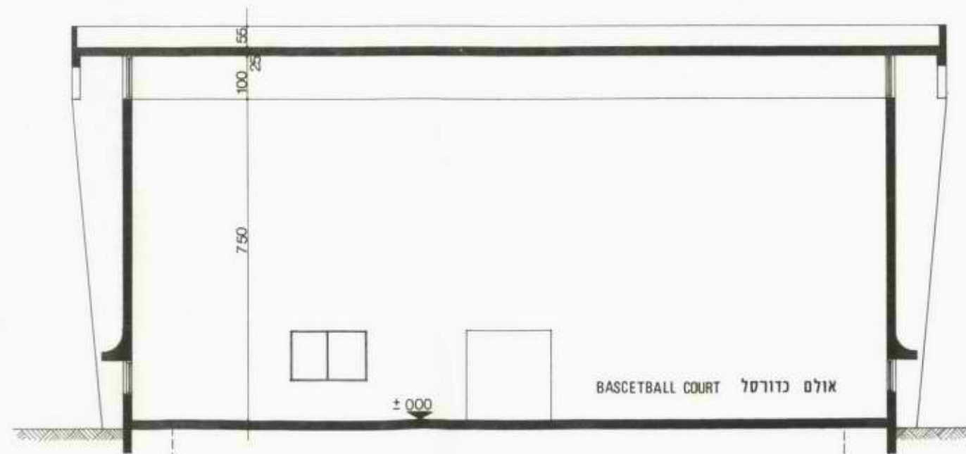
SECTION A-A חתך
