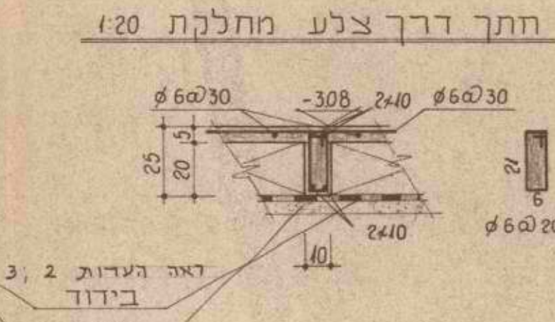
חתך דרך צלע מחלקת 1:20
