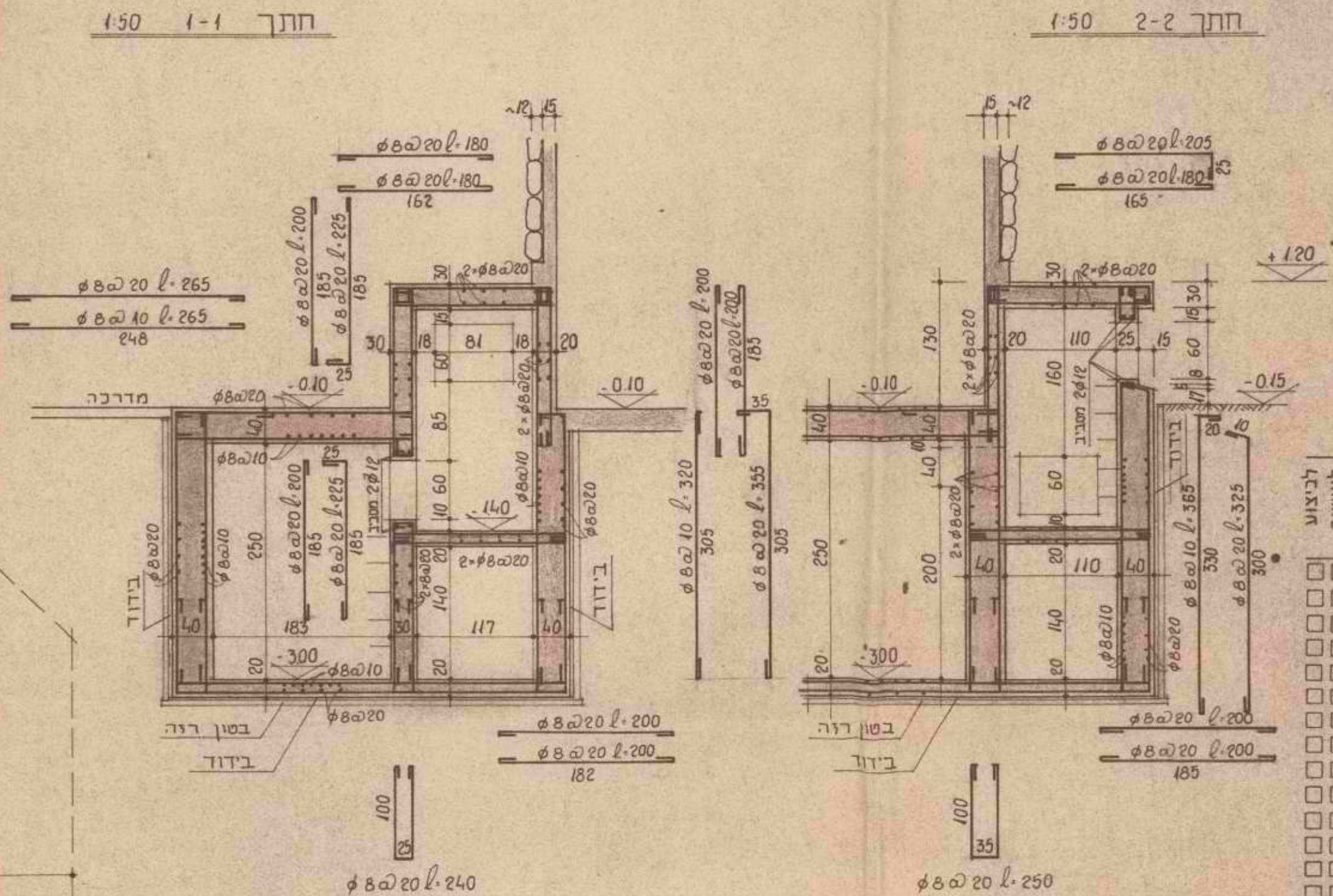
חתך 3-3 1:25
