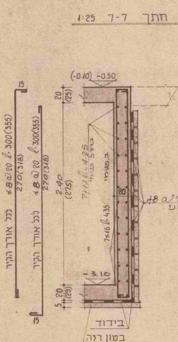
חתך 7-7 1:25
