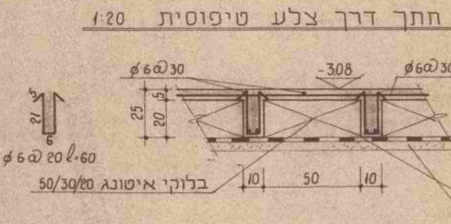
חתך דרך צלע טיפוסית 1:20
