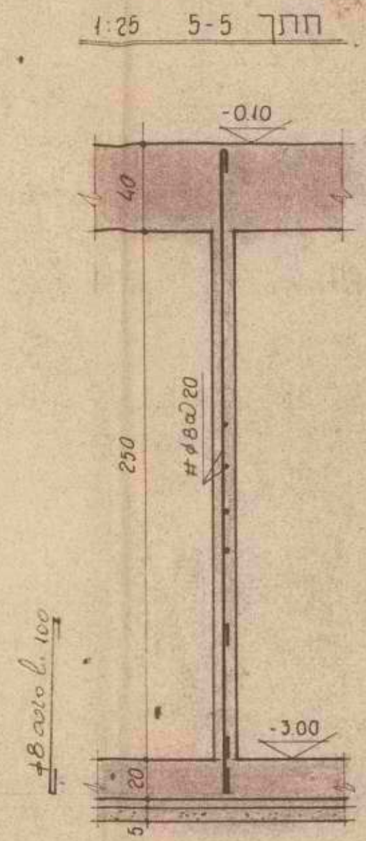
חתך 5-5 1:25
