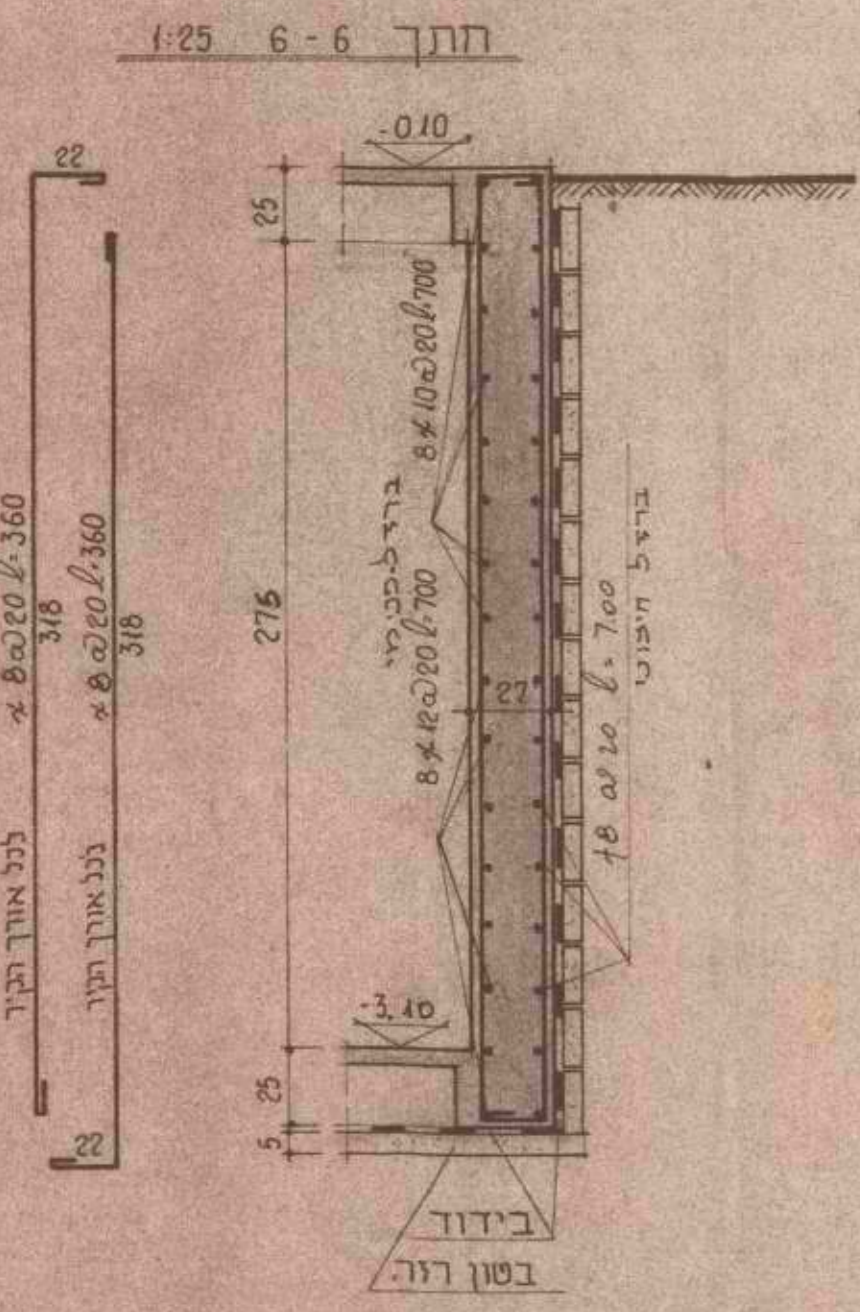
חתך 6-6 1:25
