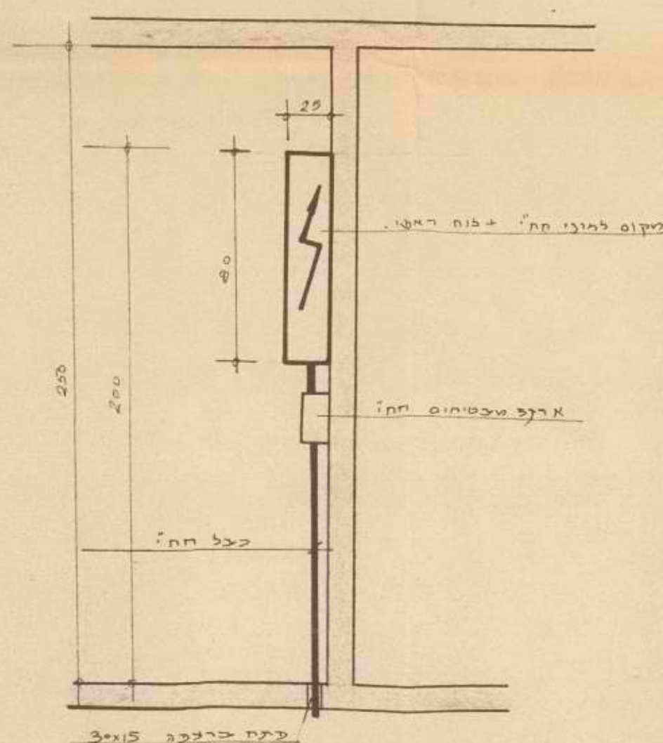
חתך 1-1 1:20 נ"ד
