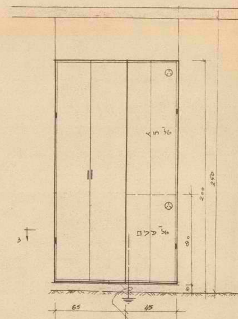
חזקה ארון 66 חוץ+ פנים ראשי וארון 55 וחמש ראשי דג"ח 1:20
