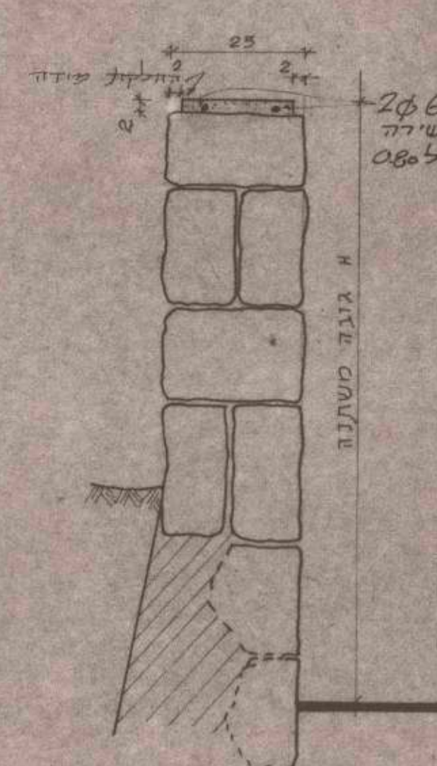
חתך ק.מ. 1:10
