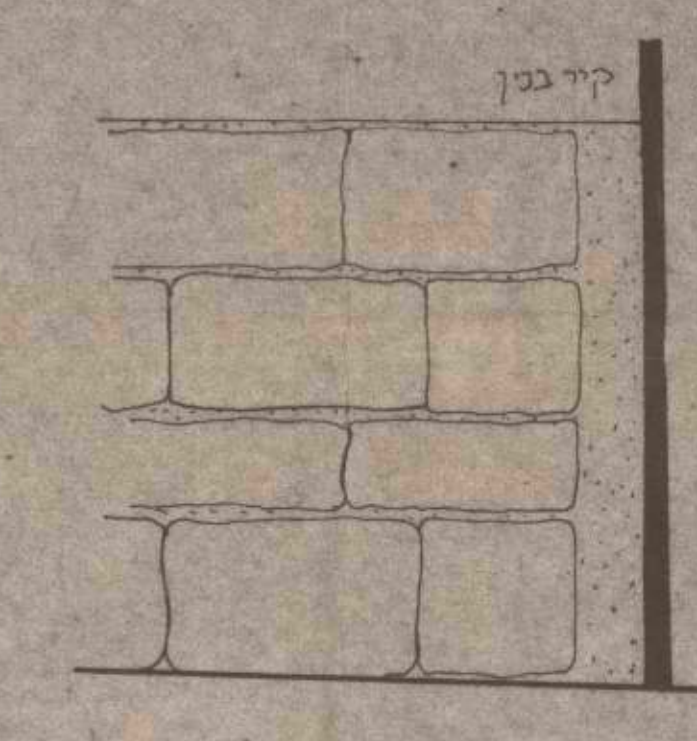
חזית ק.מ. 1:10
