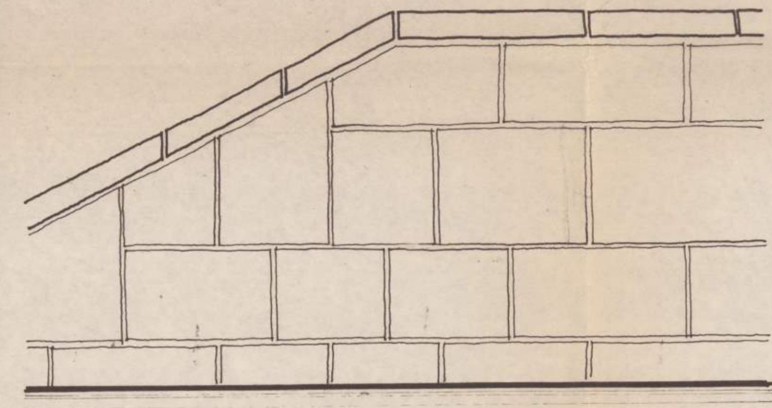
חזית קיר בשיפוע 1:10
