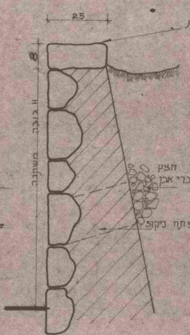
חתך ק.מ. 1:10
