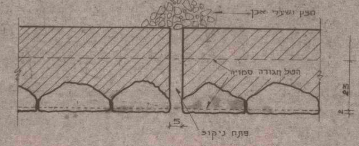
חתך ק.מ. 1:10
