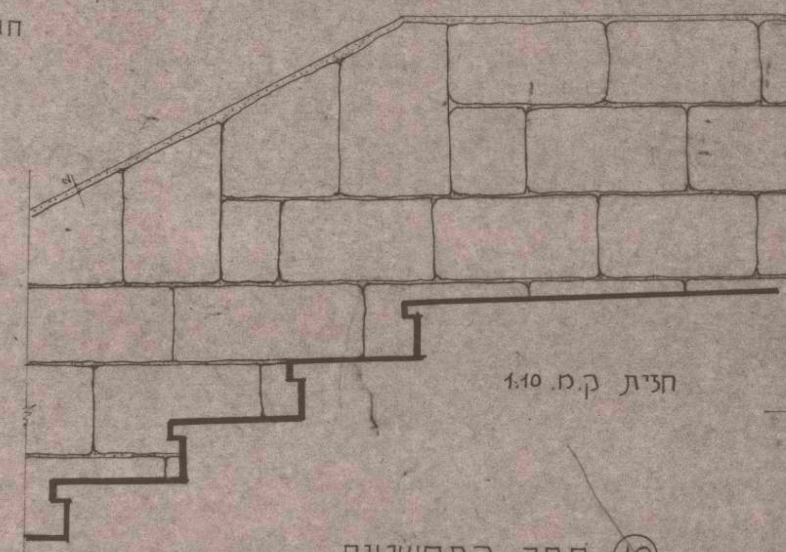
⑩ תפר התפשטות
