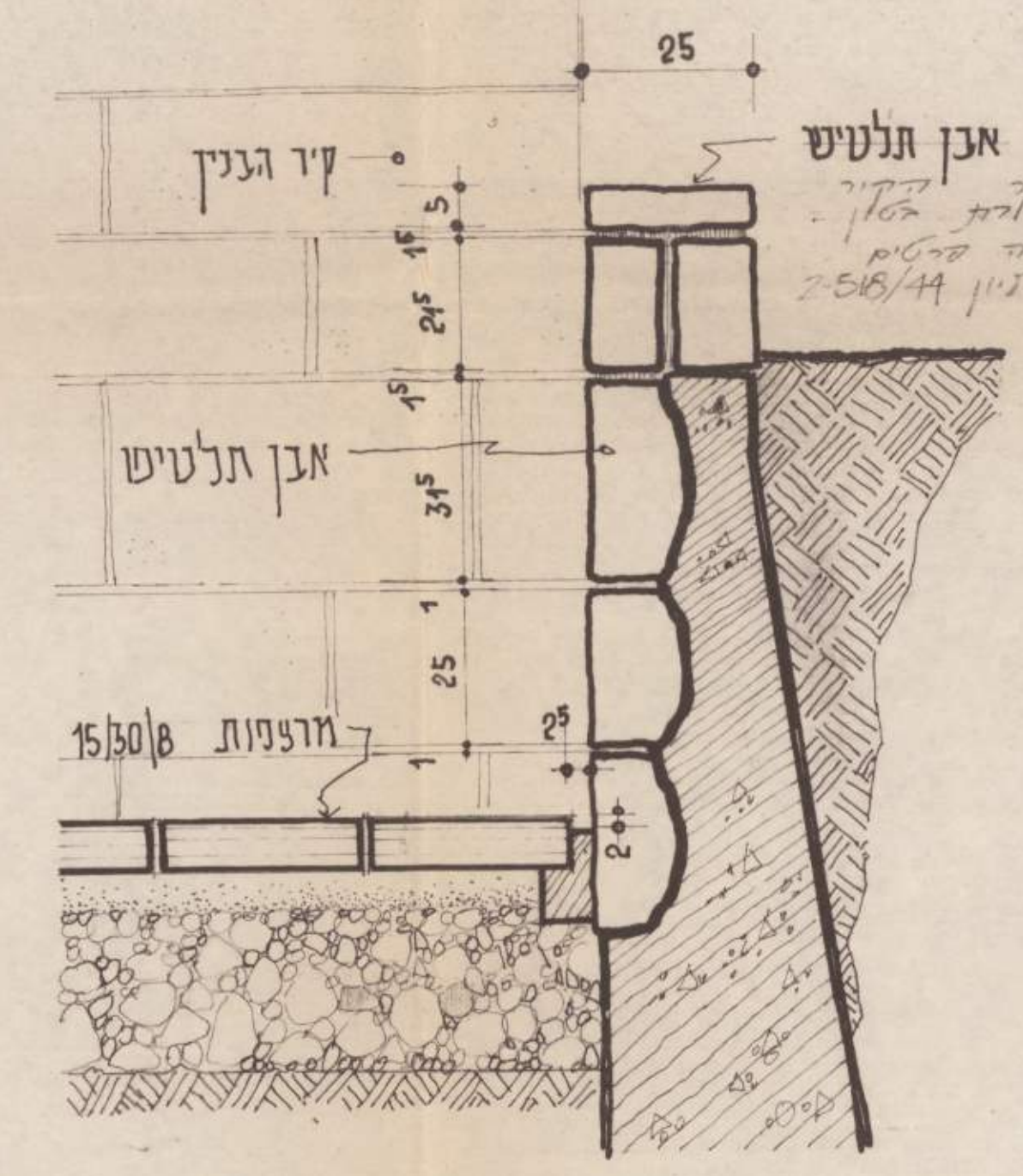
חתך אנכי 1:10
