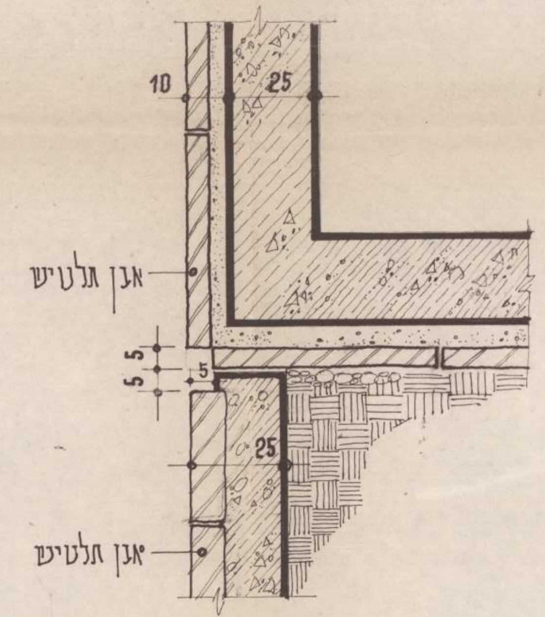
חתך אופקי 1:5
