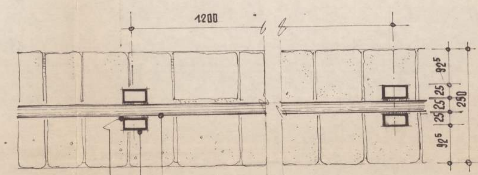
חתך אופקי 1:5
