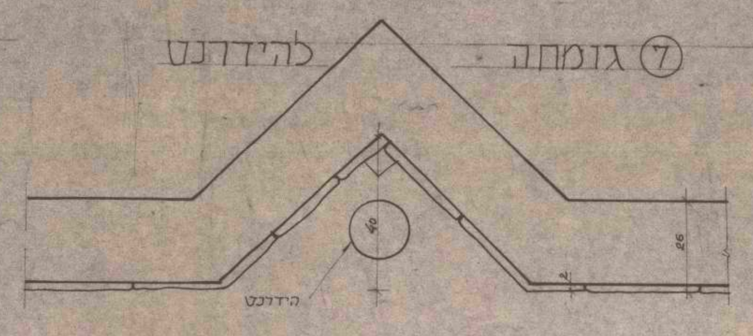
מבט על ק.מ. 1:10
