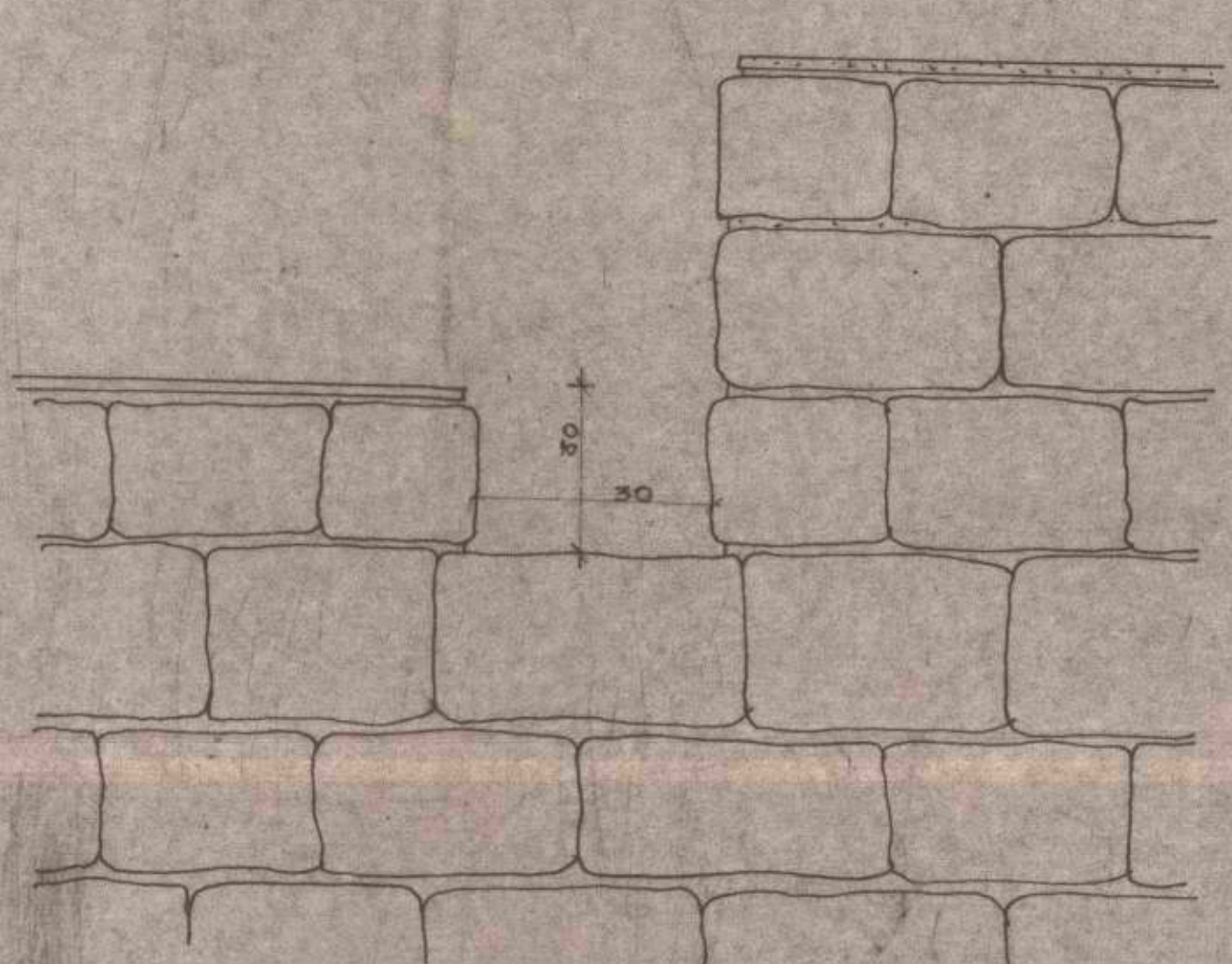
חזית ק.מ. 1:10
