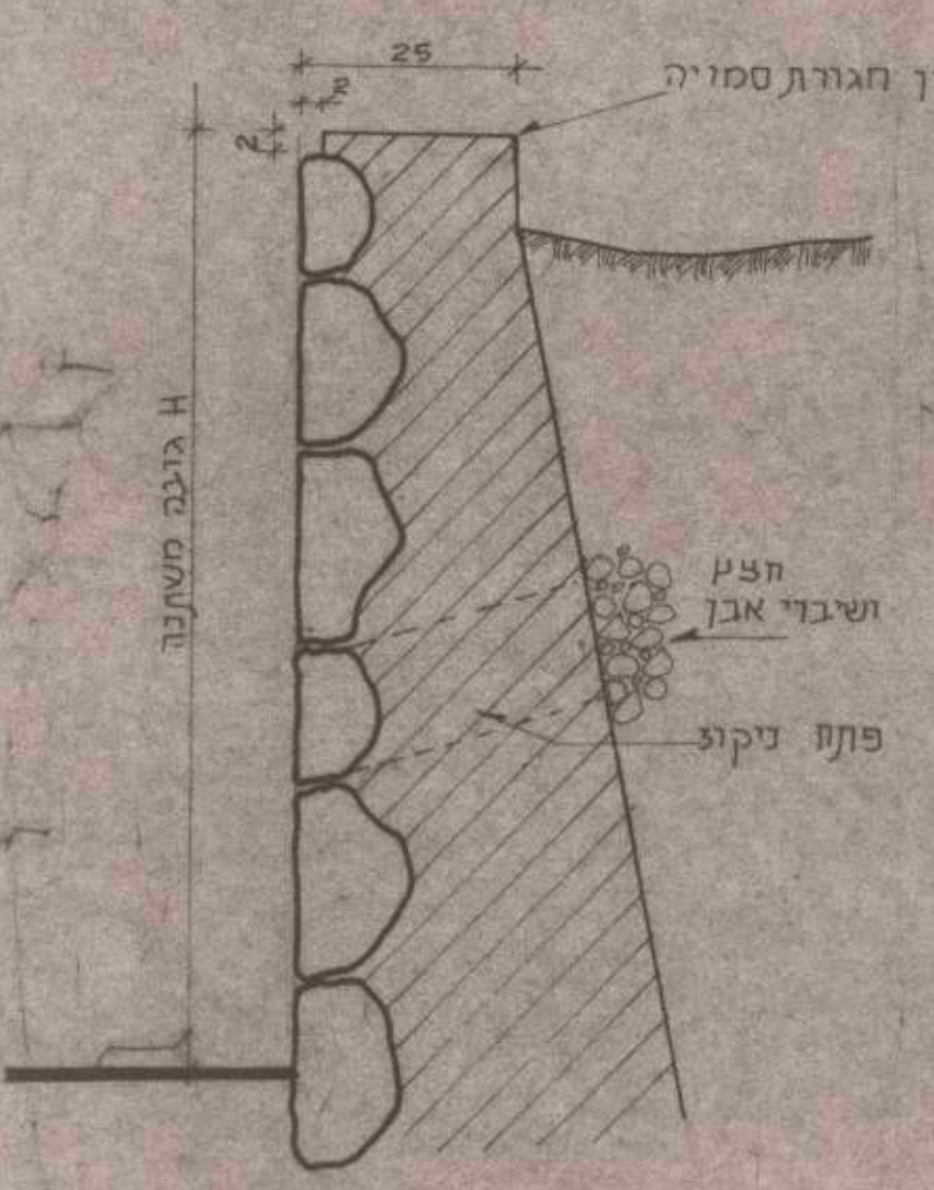
חתך ק.מ. 1:10
