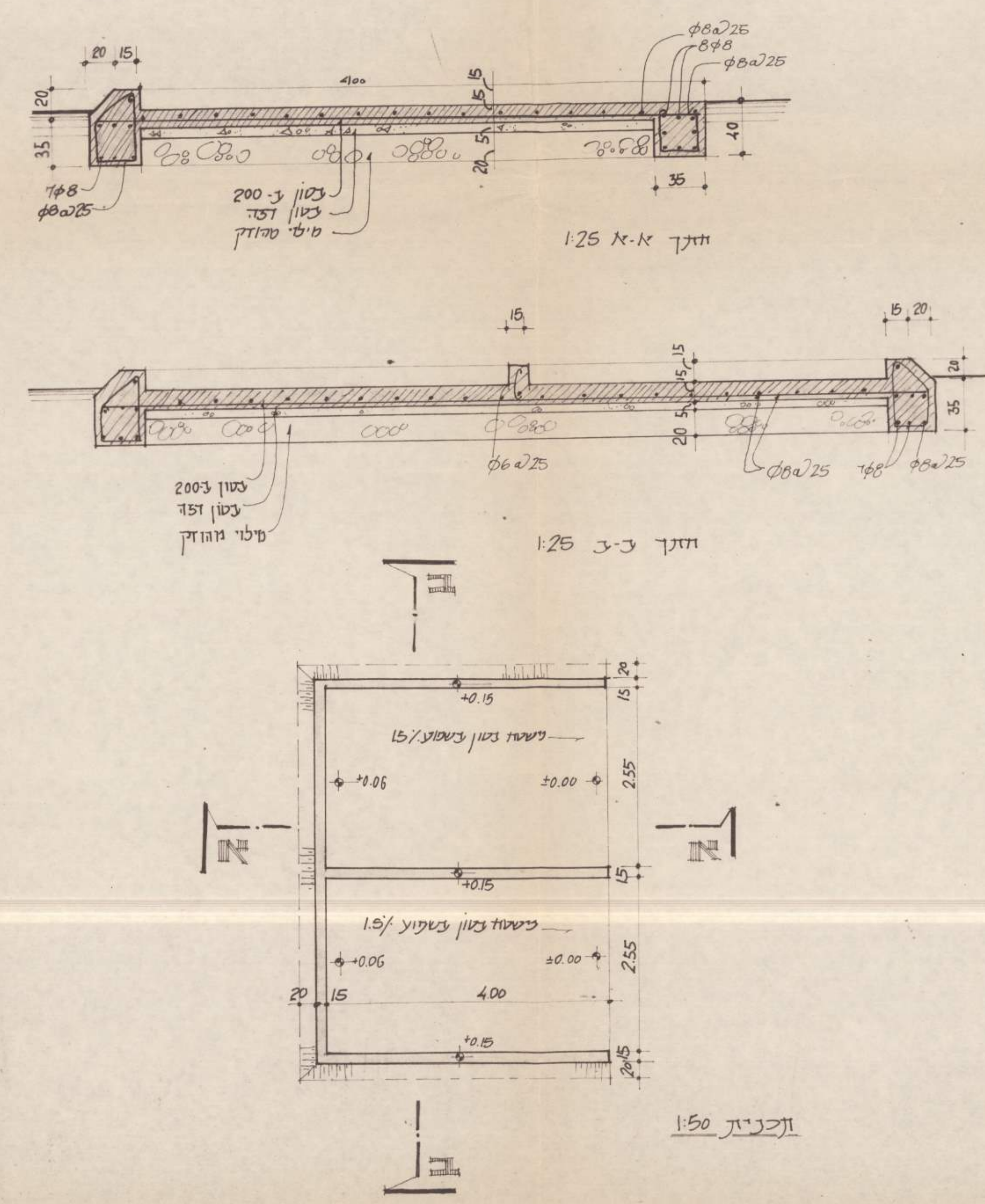
פרט משטח לעגלות אשפה
