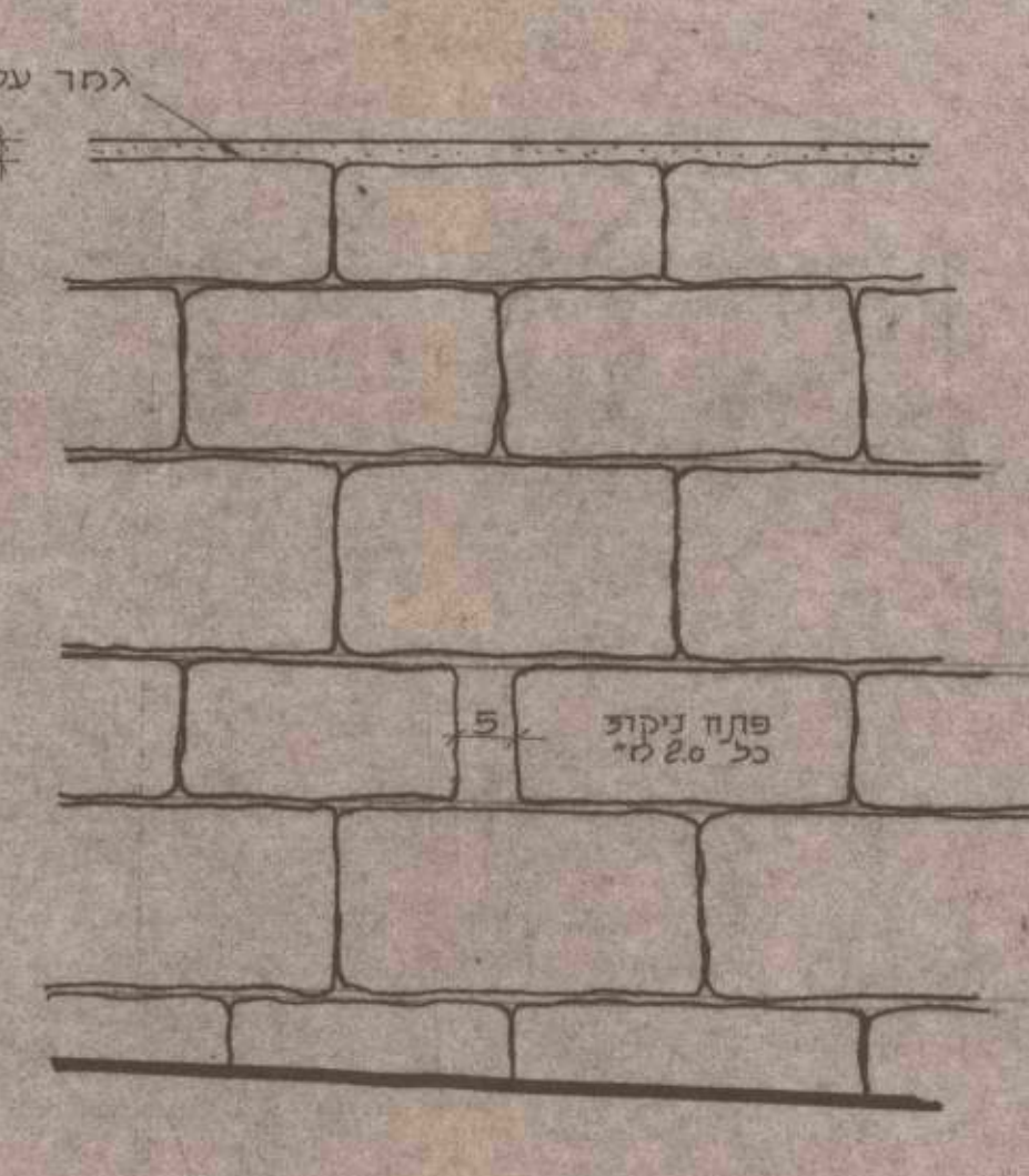
חזית ק.מ. 1:10
