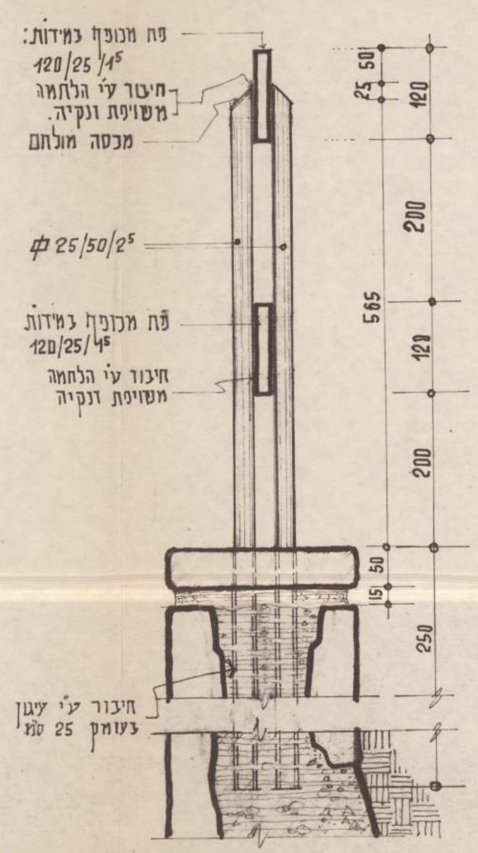
חתך אנכי 1:5
