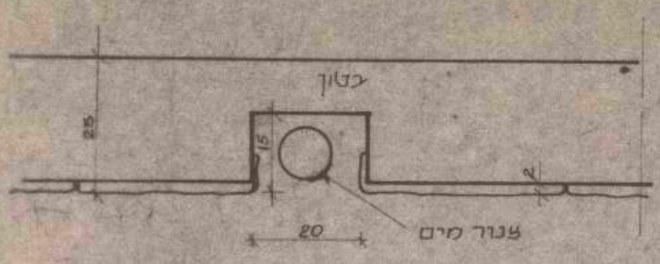
מבט על ק.מ. 1:10
