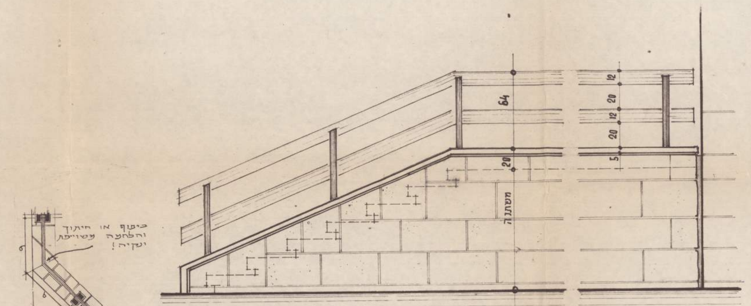
חזית מעקה לאורך מדרגות 1:20
