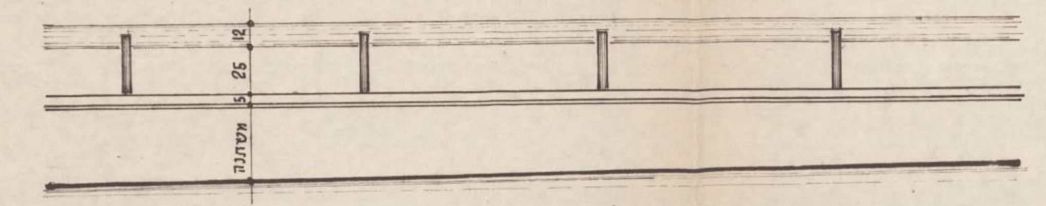
חזית קיר מעקה סביב גן ילדים 1:20
