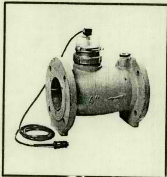
מודד WR 2" וולטמן עם פלט חשמלי לקריאה
