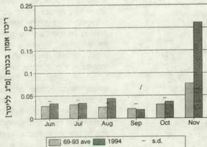
איור 7: ריכוזי אמון (מ"ג לליטר) באפילימניון (ממוצע לעומקים 0 עד 10 מ') בכנרת. השוואה בין חודשי קיץ-סתיו 1994 והממוצע הרב-שנתי (1969 עד 1993) לאותם חודשים. s.d. = סטיית תקן (נתונים: ע. נשרי, מ. שליכטר, ט. ברמן).
