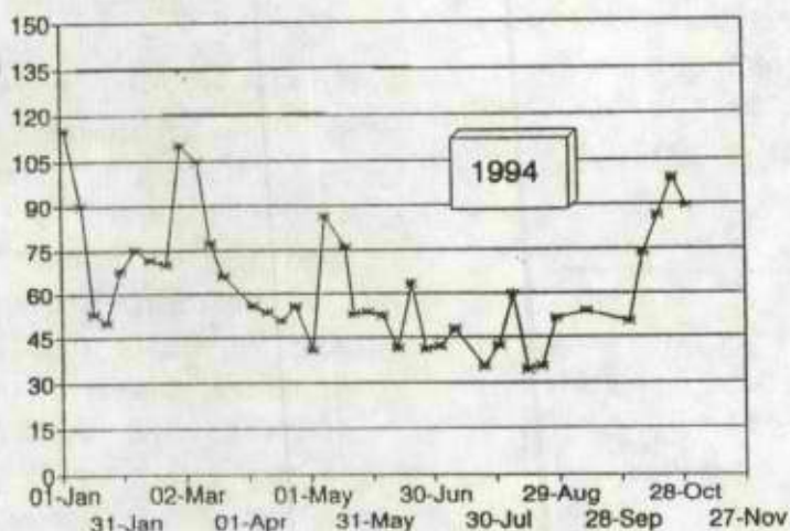
יחס חנקן כללי לזרחן כללי
