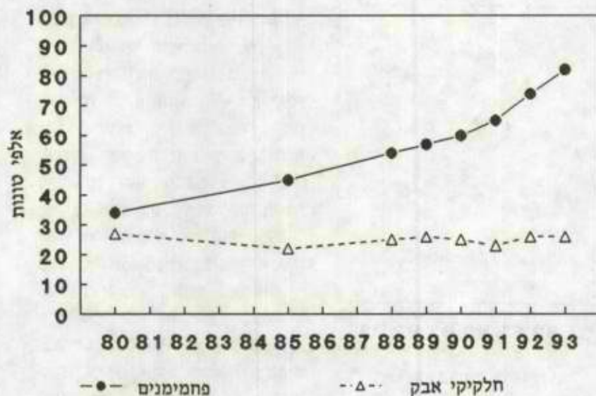
איור 4: פליטות שנתיות של חלקיקי אבק ופחמימנים בישראל בשנים 1980-1993.
