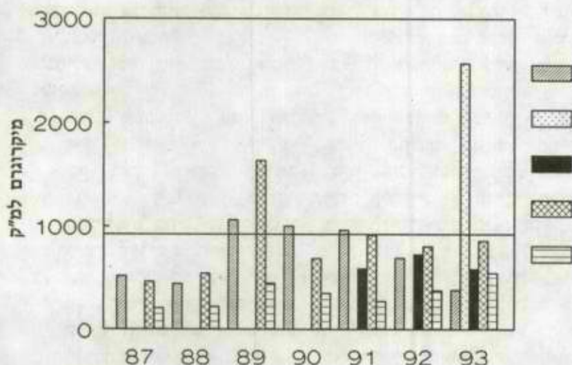
איור 7: ריכוזי תחמוצות חנקן באוויר (ערך חציישעתי מירבי). הקו מסמן את התקן המוחלט (940 מיקרוגרם למ"ק).
