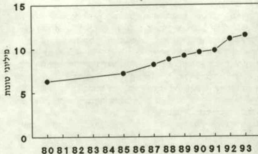
איור 1: פליטה שנתית של פחמן דו-חמצני בישראל בשנים 1980-1993.
