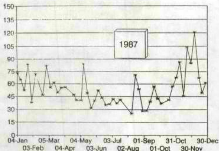
יחס חנקן כללי לזרחן כללי
