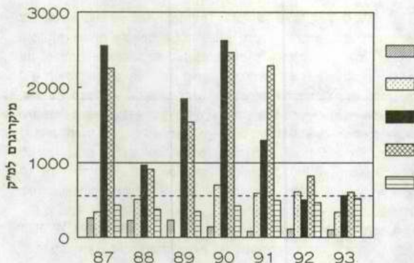
איור 6: ריכוזי גופרית דו-חמצנית באוויר (ערך חציישעתי מירבי). הקו המלא - תקן מוחלט שאין לחרוג ממנו; הקו המרוסק - תקן סטטיסטי 99.75% (ראה הסבר בגוף המאמר).
