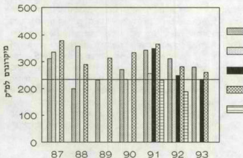
איור 8: ריכוזי אוזון באוויר (ערך חציישעתי מירבי). הקו מסמן את התקן המוחלט (230 מיקרוגרם למ"ק).
