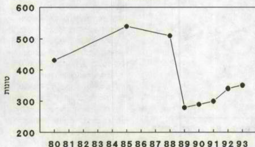
איור 5: פליטה שנתית לאוויר של עופרת בישראל בשנים 1980-1993.
