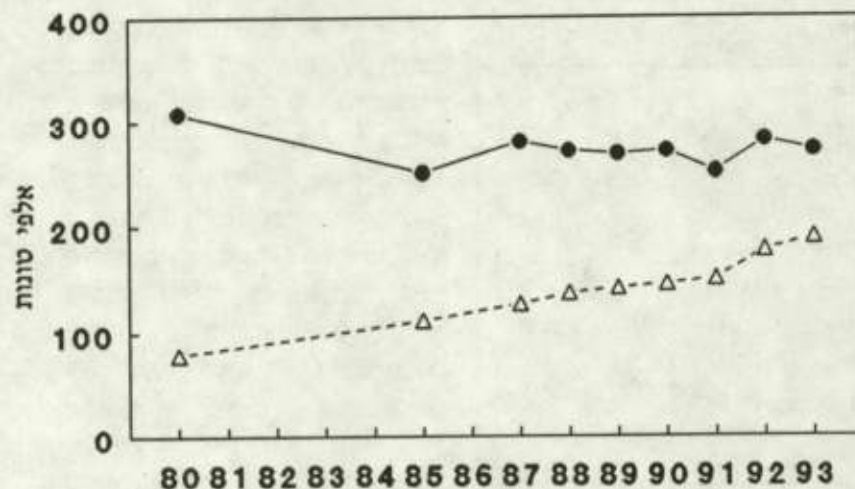
איור 3: פליטות שנתיות של תחמוצות גופרית ותחמוצות חנקן בישראל בשנים 1980-1993.
