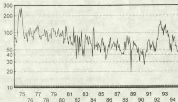
יחס חנקן כללי לזרחן כללי באפילימניון
