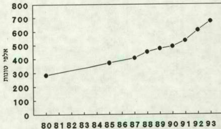
איור 2: פליטה שנתית של פחמן חד-חמצני בישראל בשנים 1980-1993.
