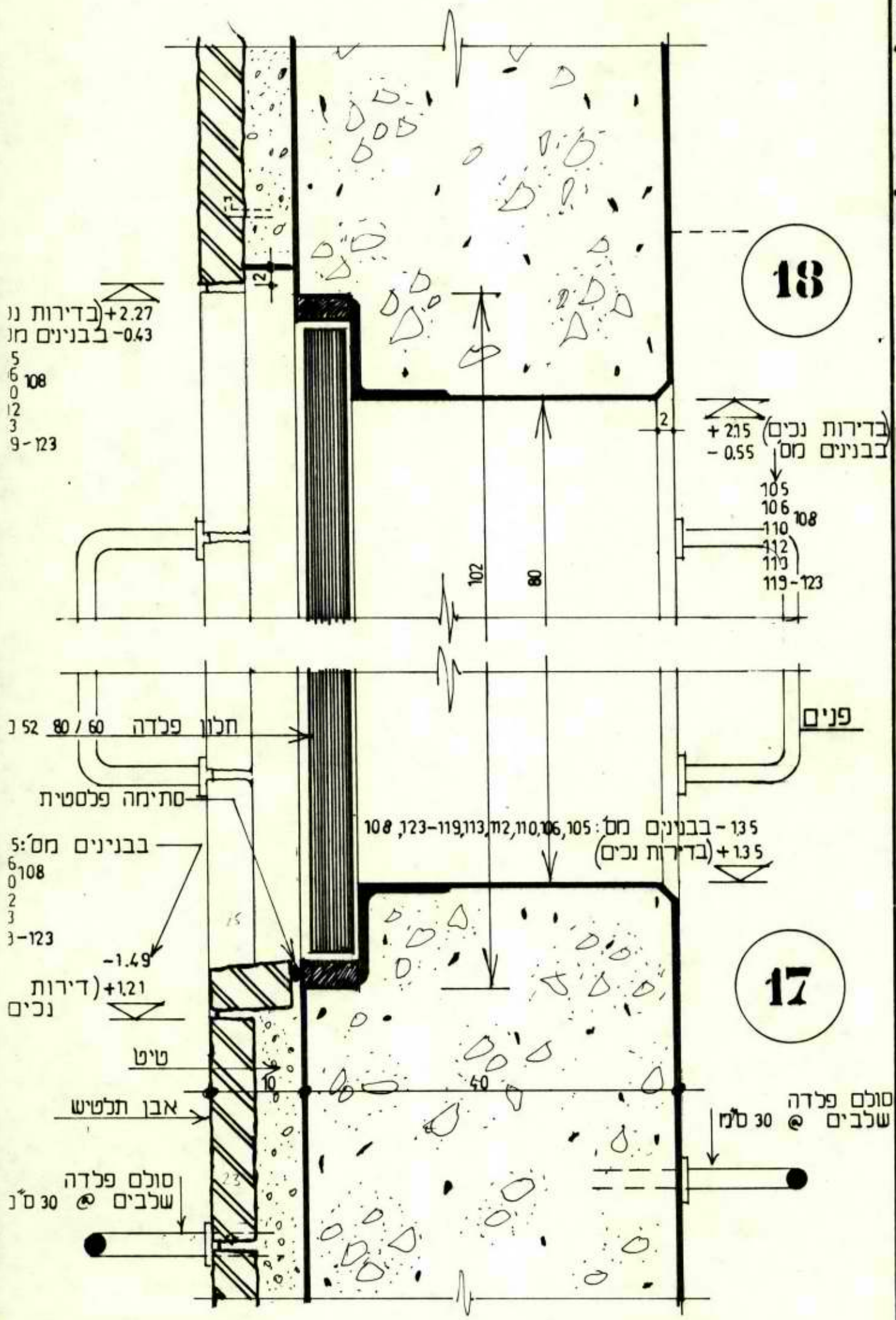
יציאת חירום (על קרקעית) פרט אנכי
