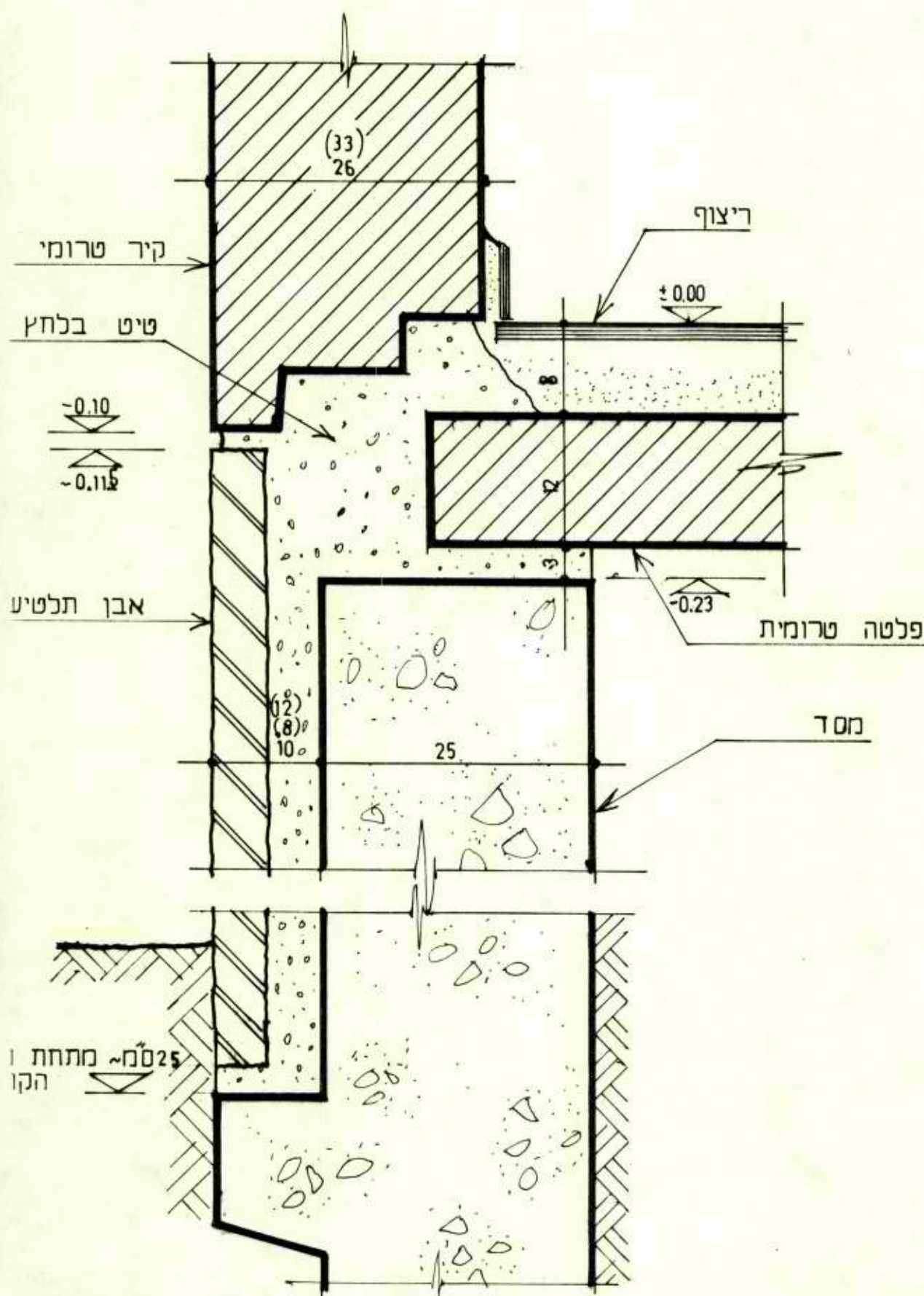
פרט אנכי אופיני של מסד-קיר טרומי
