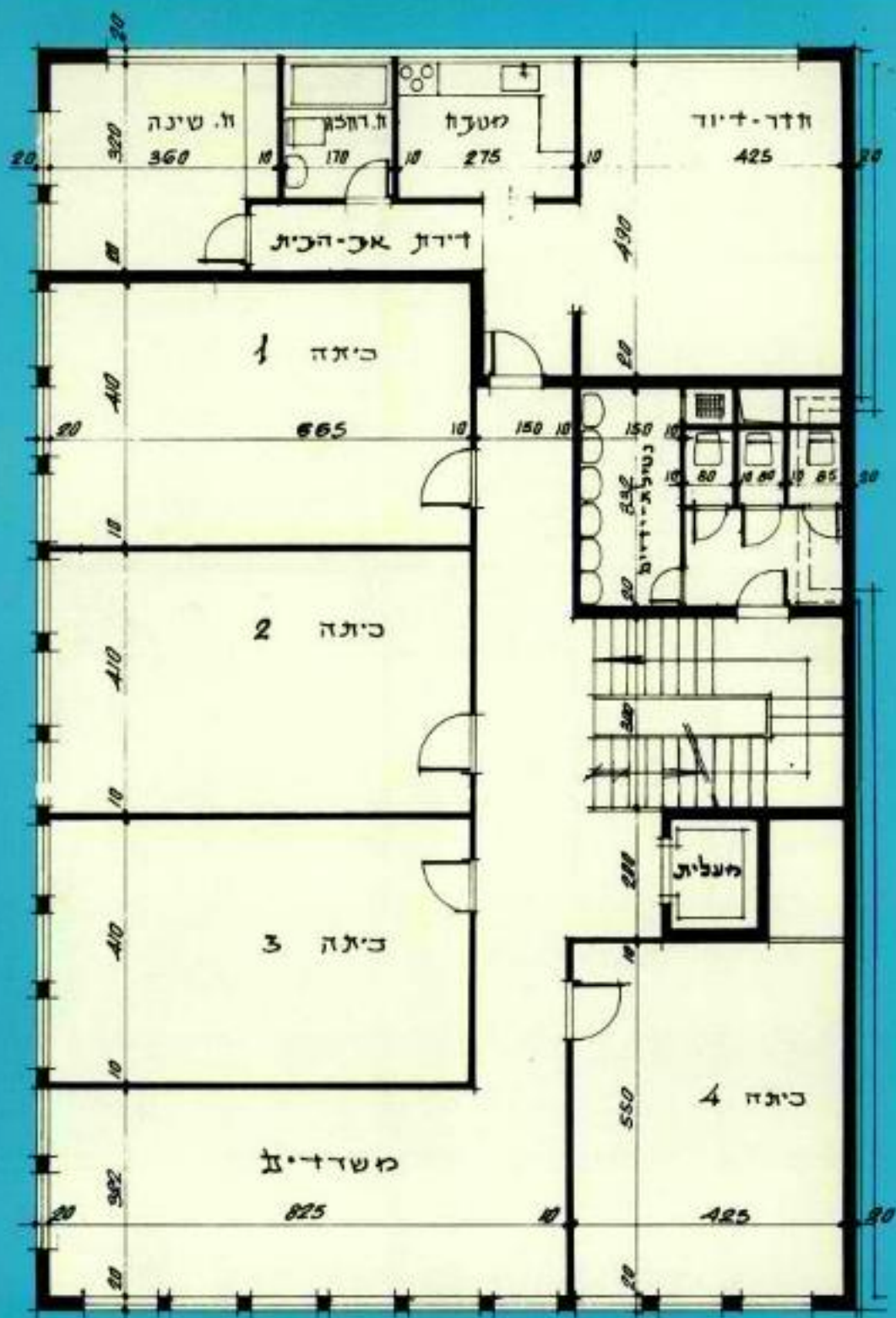
תכנית קומה א' כיתות לימוד ומשרדי ההנהלה
