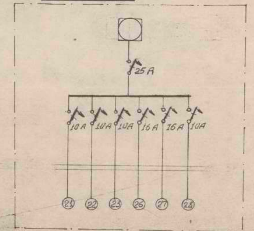
סכמה לדירה
