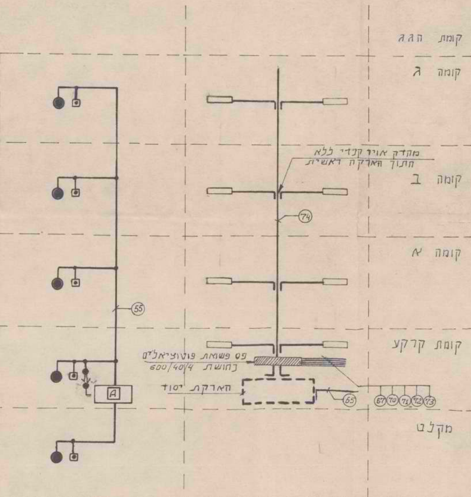
VERTICAL DIAGRAM OF STAIRS CASE סכמה למאור חדר מדרגות
