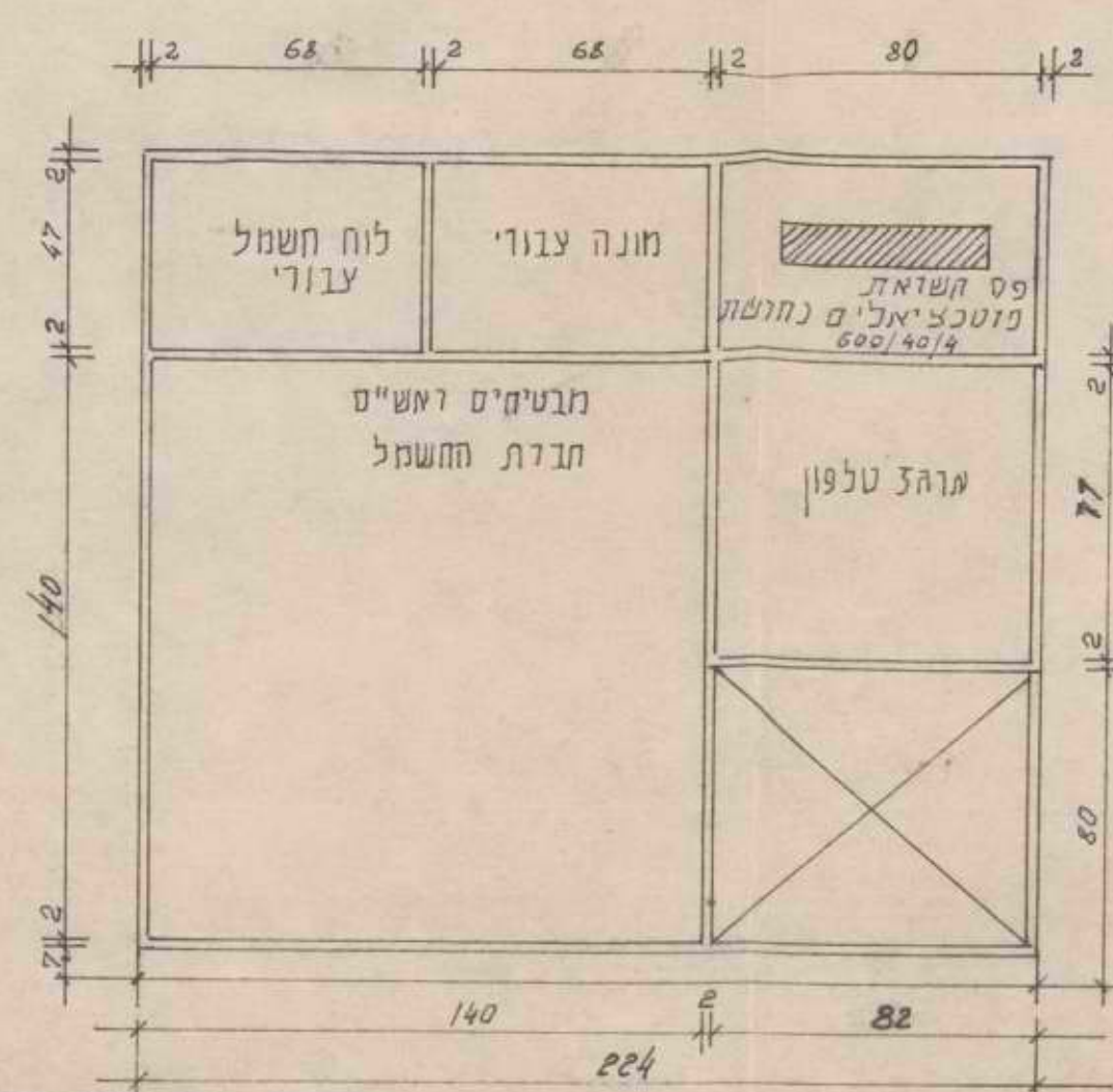
MAIN DISTRIBUTION BOARD לוח חשמל ראשי
