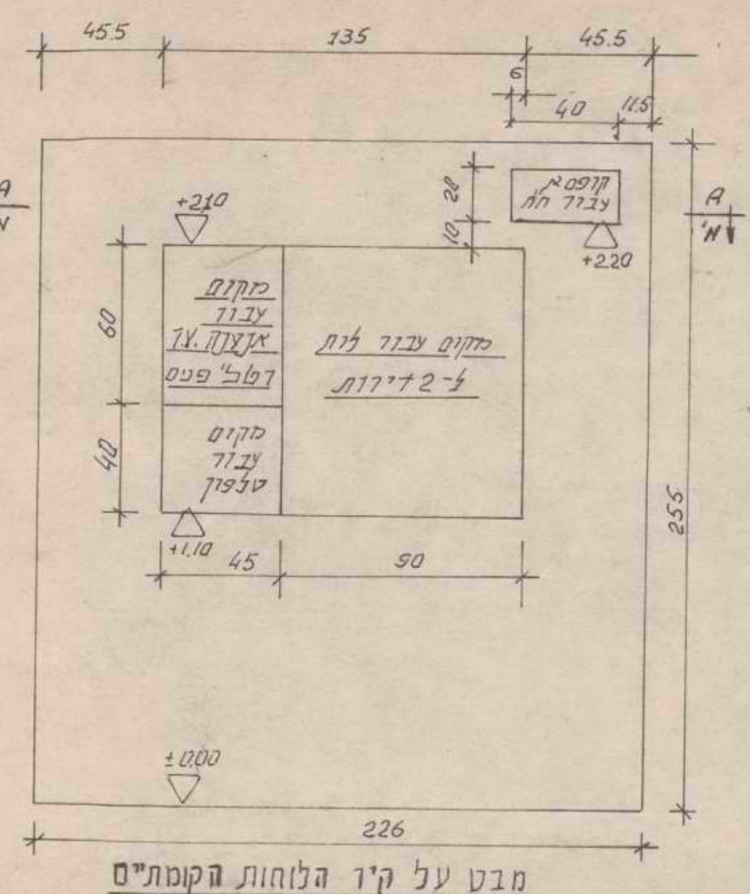
מבט על קווי הלוחות הקומתיים
