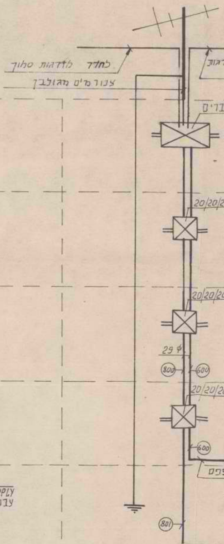
VERTICAL DIAGRAM OF T.V. סכמה לתוכנית טלוויזיה ולטלפון פנים
