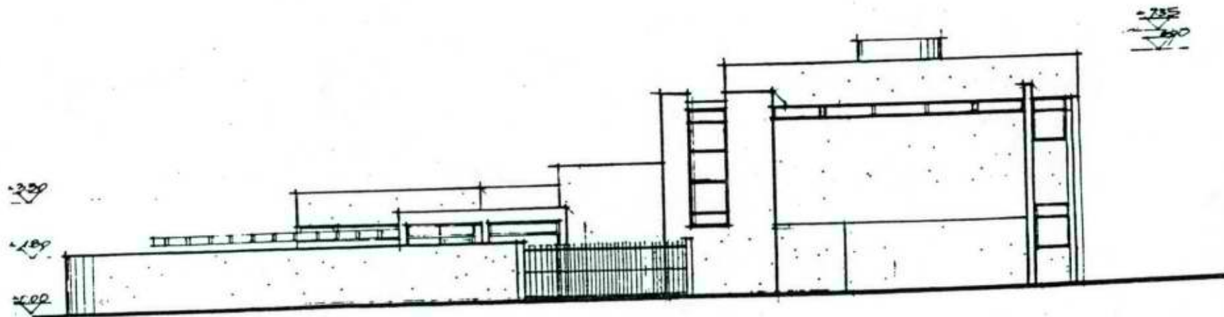
חזית דרומית
