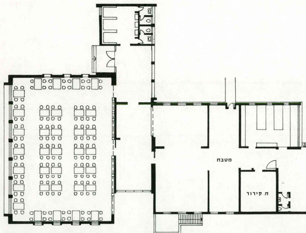
ח. אוכל ומטבח תכנית
