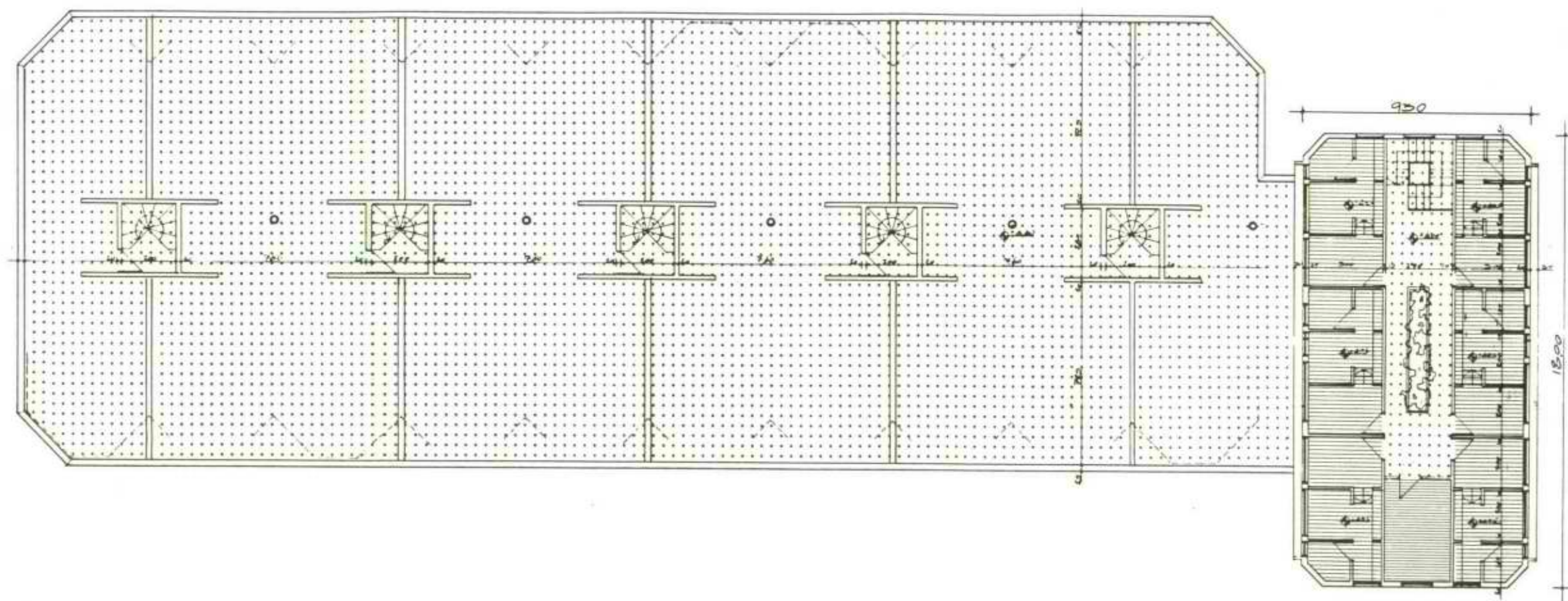
תכנית קומה שלושית / גג THIRD FLOOR & ROOF PLAN
